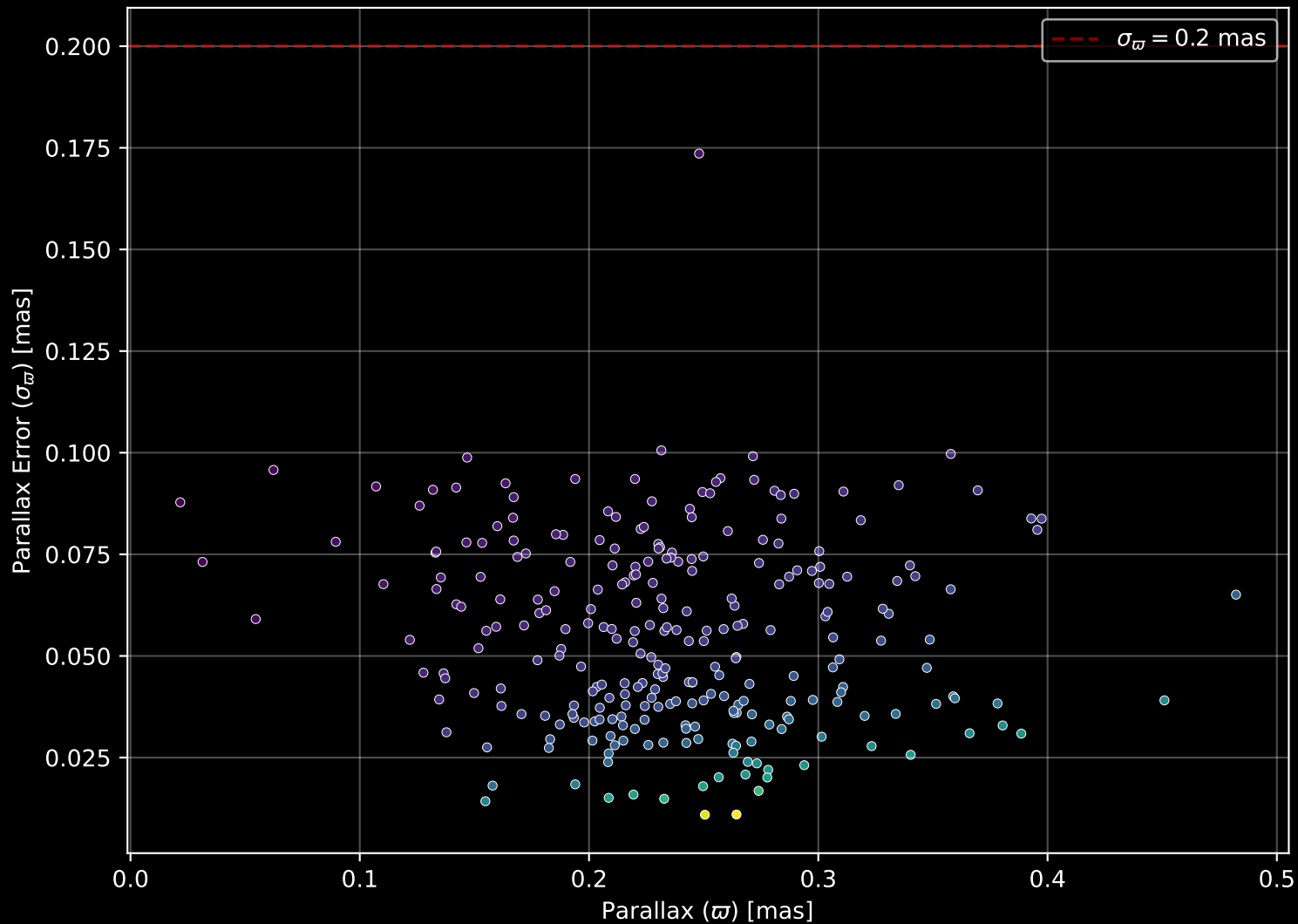
Gaia Cluster: [Ruprecht_28] Parallax Quality (n= 270)
