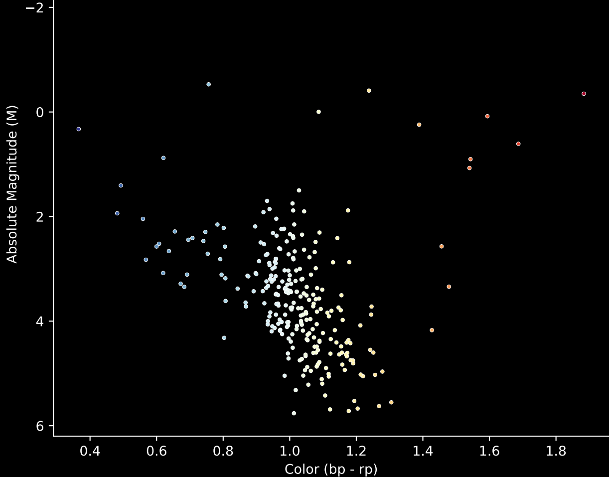
Gaia Cluster: [Ruprecht_28] Stars (n= 270) Hertzsprung-Russel Diagram
