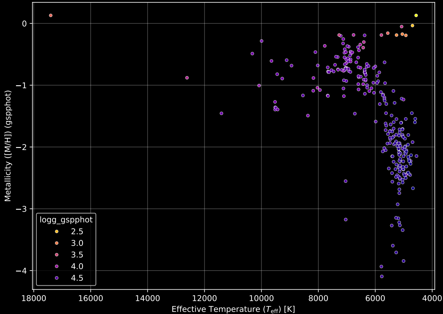
Gaia Cluster: [Ruprecht_28] Stellar Population Parameters (n= 270)
