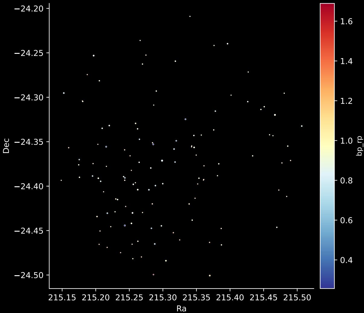
Gaia Cluster: [Ruprecht_29] Stars: 120
