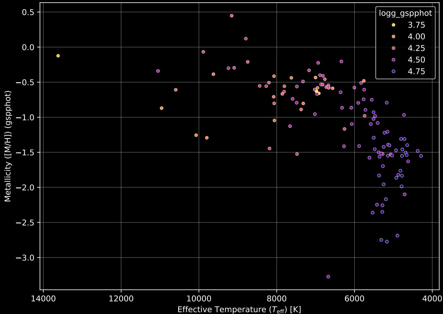
Gaia Cluster: [Ruprecht_29] Stellar Population Parameters (n= 120)
