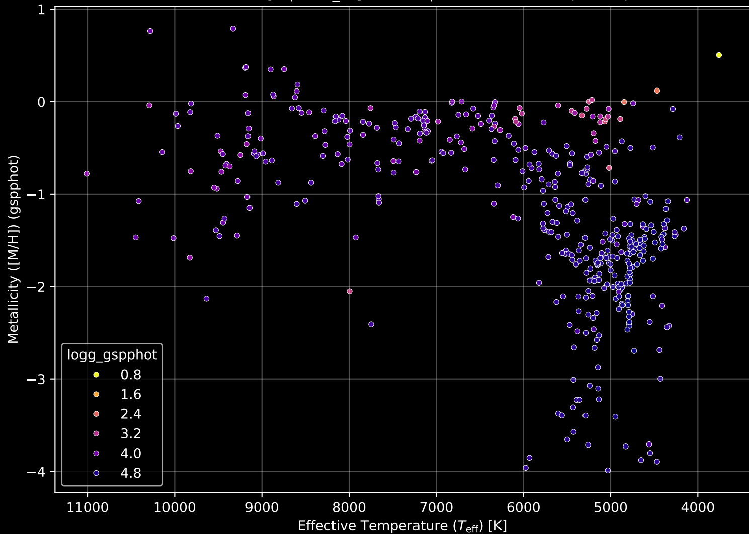
Gaia Cluster: [Ruprecht_34] Stellar Population Parameters (n= 438)
