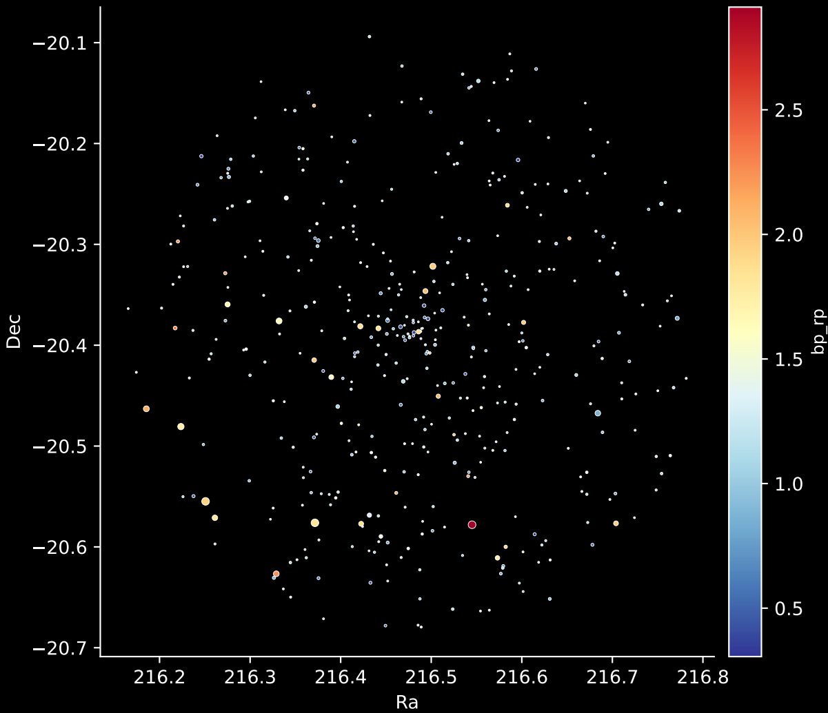
Gaia Cluster: [Ruprecht_34] Stars: 438
