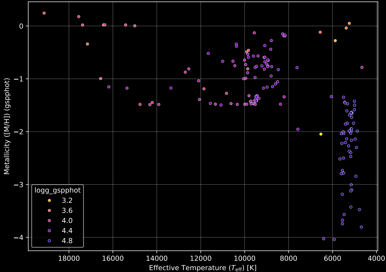
Gaia Cluster: [Ruprecht_35] Stellar Population Parameters (n= 158)
