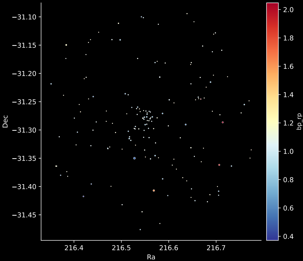
Gaia Cluster: [Ruprecht_35] Stars: 158
