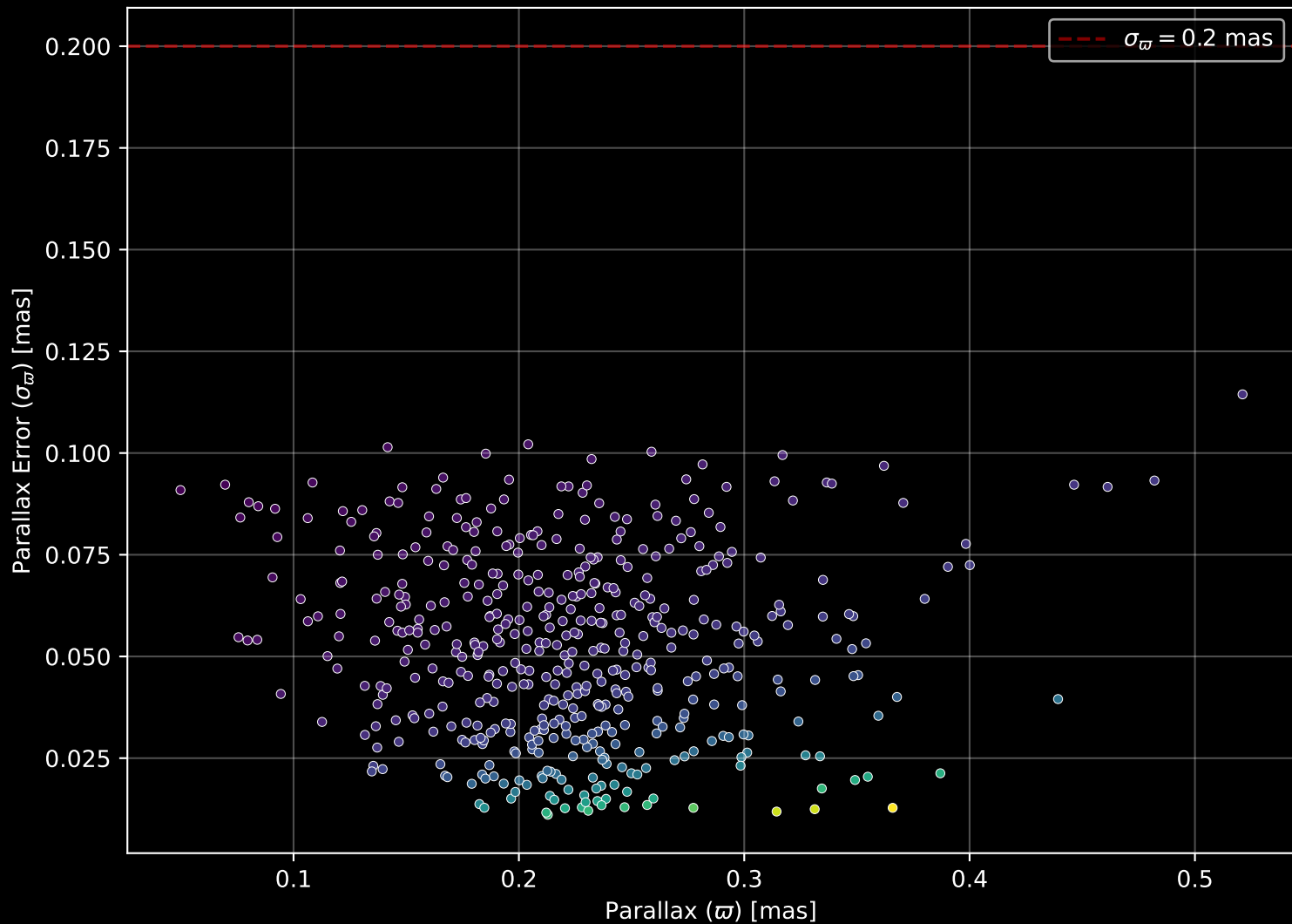
Gaia Cluster: [Ruprecht_41] Parallax Quality (n= 472)
