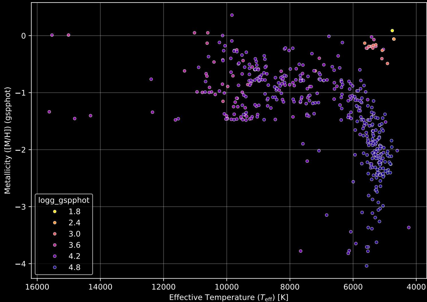
Gaia Cluster: [Ruprecht_41] Stellar Population Parameters (n= 472)
