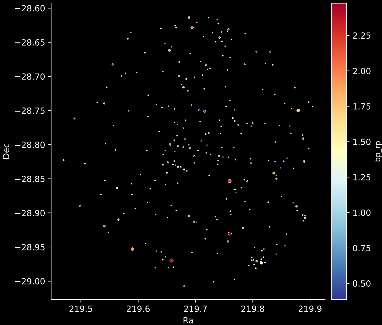
Gaia Cluster: [Ruprecht_43] Stars: 253
