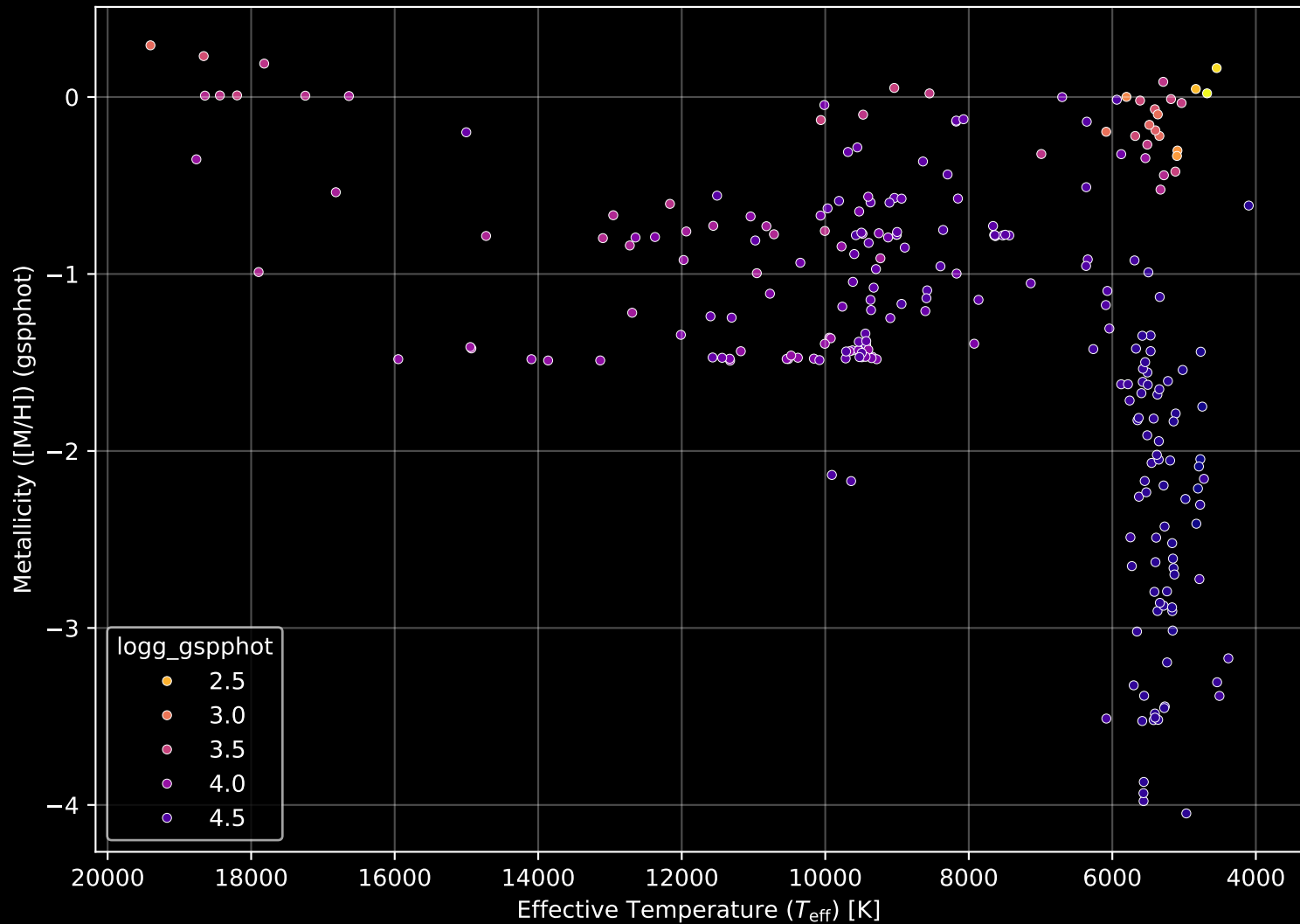
Gaia Cluster: [Ruprecht_43] Stellar Population Parameters (n= 253)
