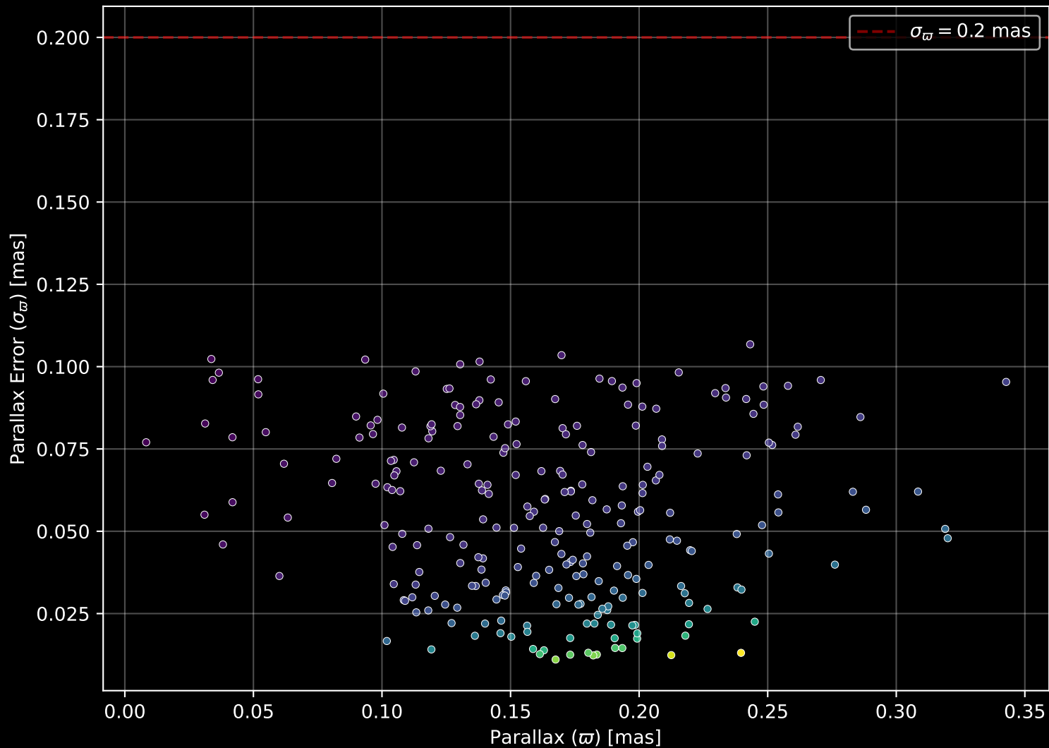
Gaia Cluster: [Ruprecht_43] Parallax Quality (n= 253)
