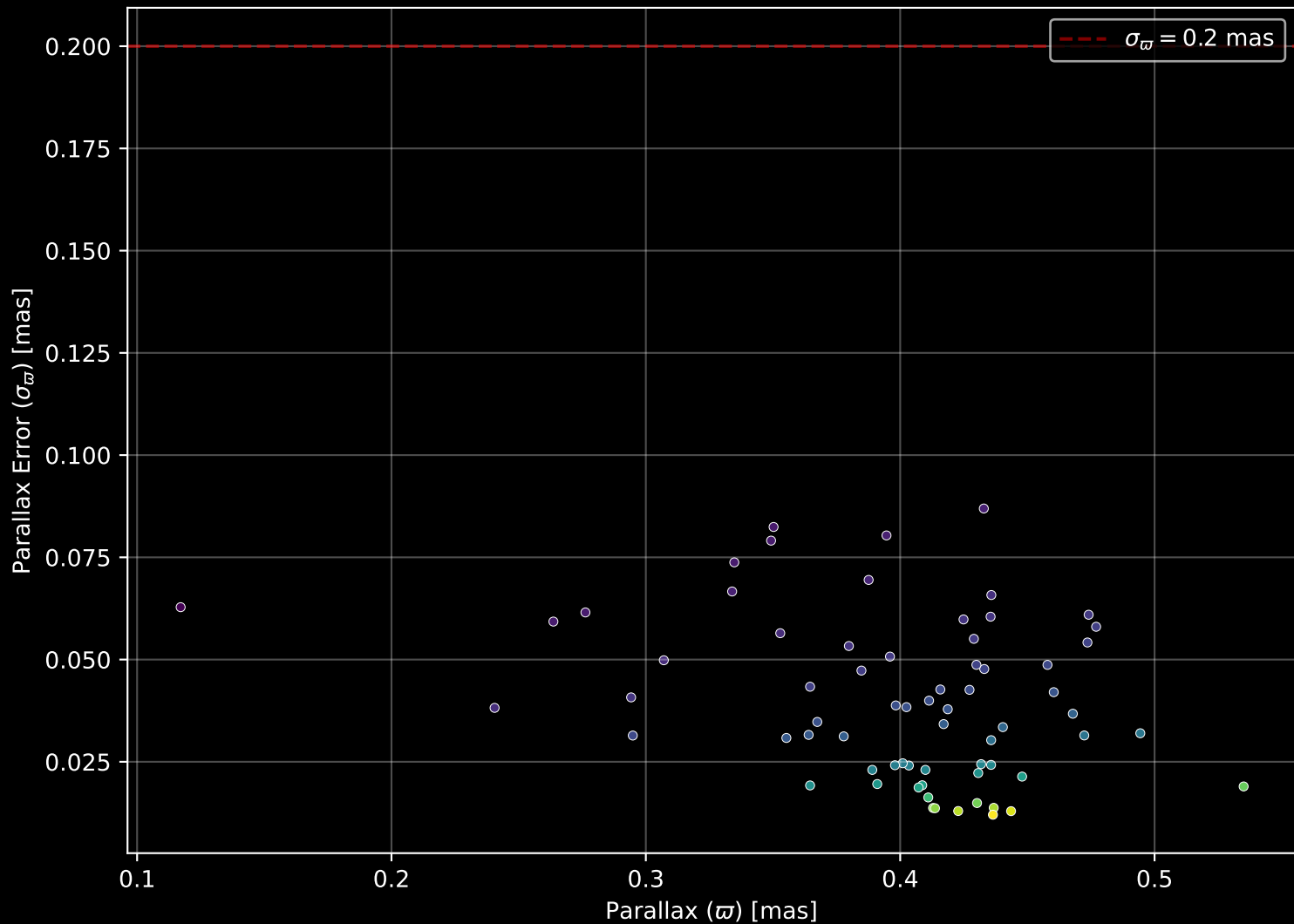
Gaia Cluster: [Ruprecht_50] Parallax Quality (n= 68)
