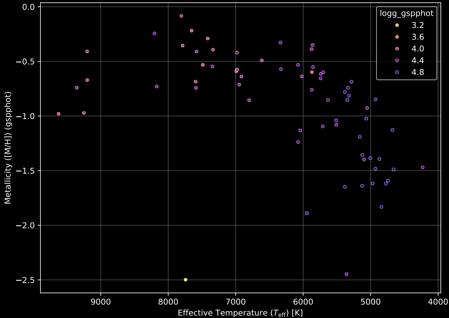
Gaia Cluster: [Ruprecht_50] Stellar Population Parameters (n= 68)
