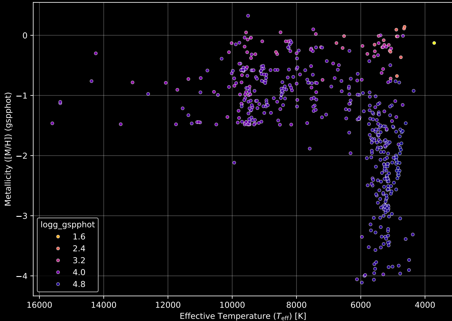
Gaia Cluster: [Ruprecht_54] Stellar Population Parameters (n= 505)
