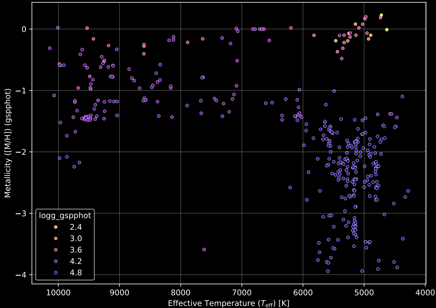
Gaia Cluster: [Ruprecht_63] Stellar Population Parameters (n= 361)
