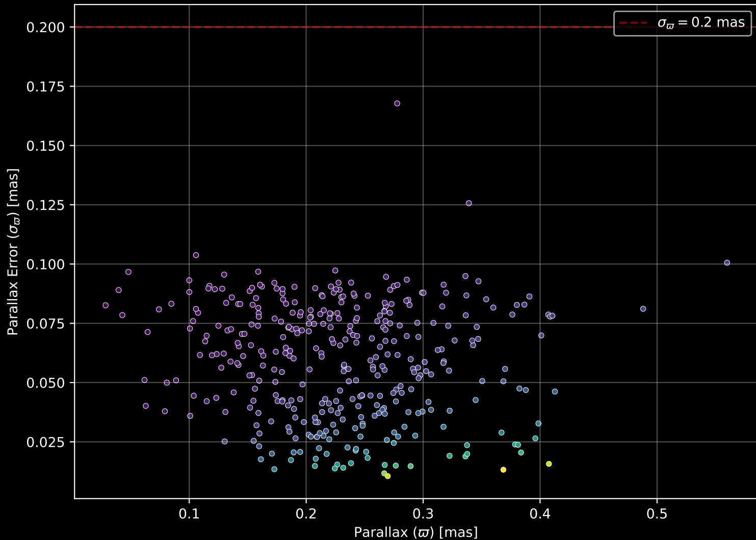
Gaia Cluster: [Ruprecht_63] Parallax Quality (n= 361)
