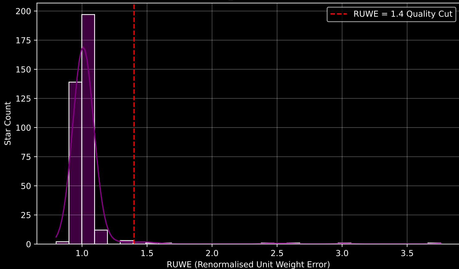
Gaia Cluster: [Ruprecht_63] RUWE Distribution (n= 361)
