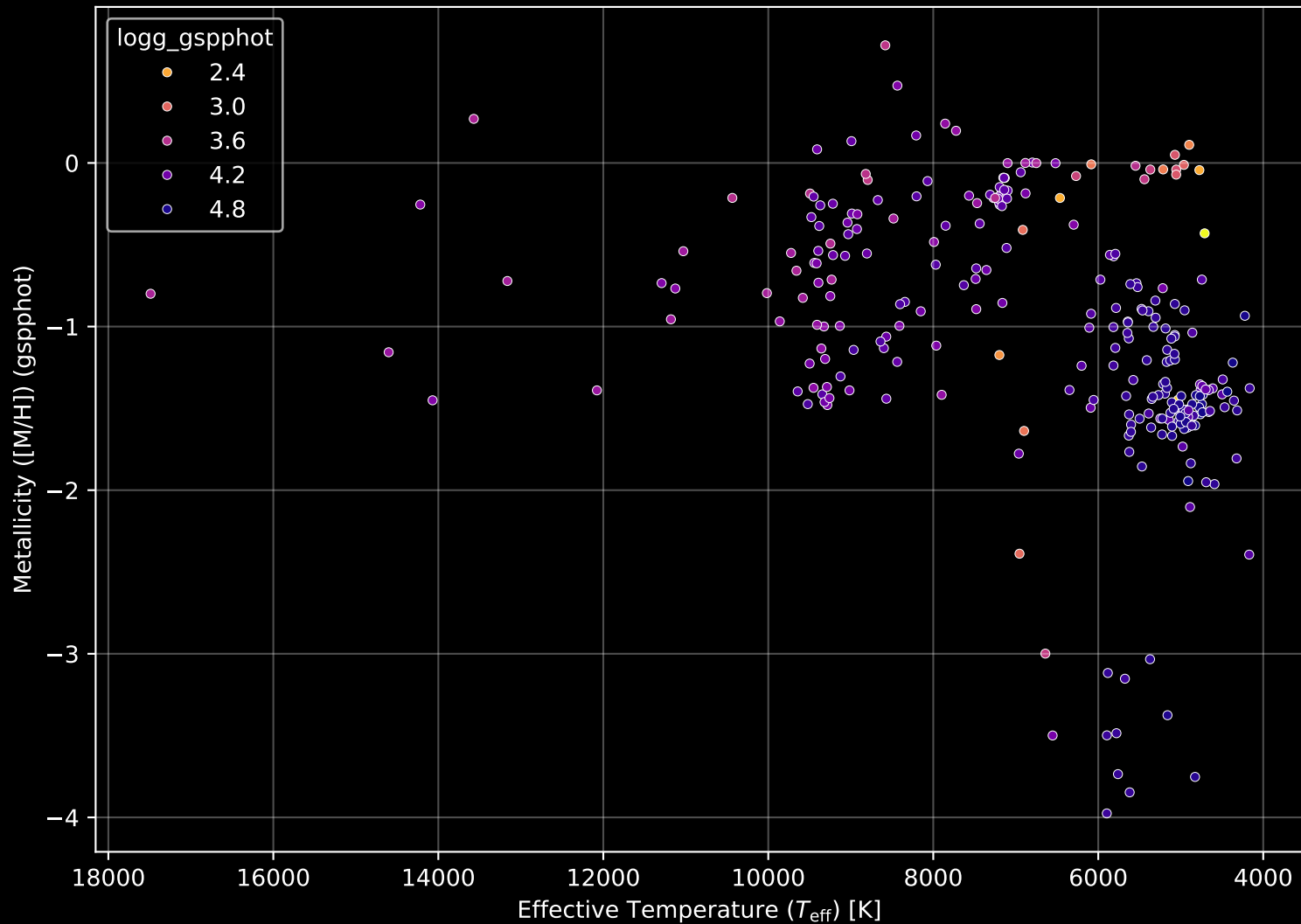
Gaia Cluster: [Ruprecht_65] Stellar Population Parameters (n= 272)
