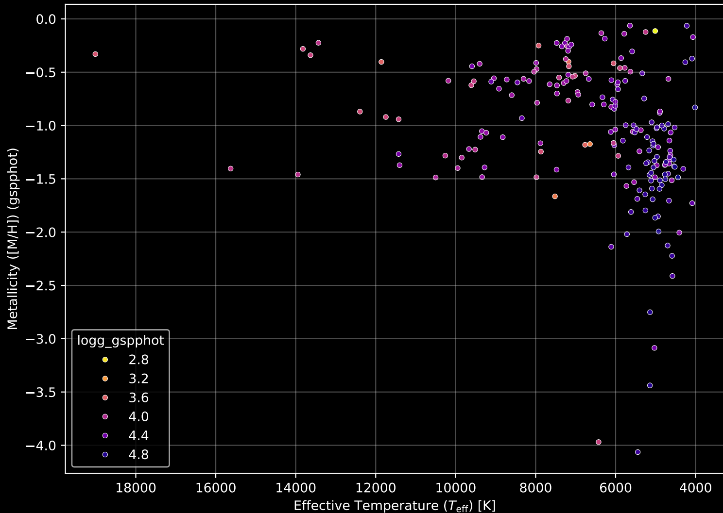
Gaia Cluster: [Ruprecht_71] Stellar Population Parameters (n= 195)
