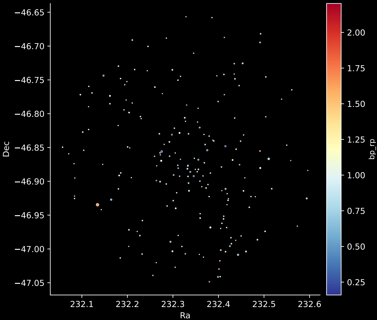
Gaia Cluster: [Ruprecht_71] Stars: 195
