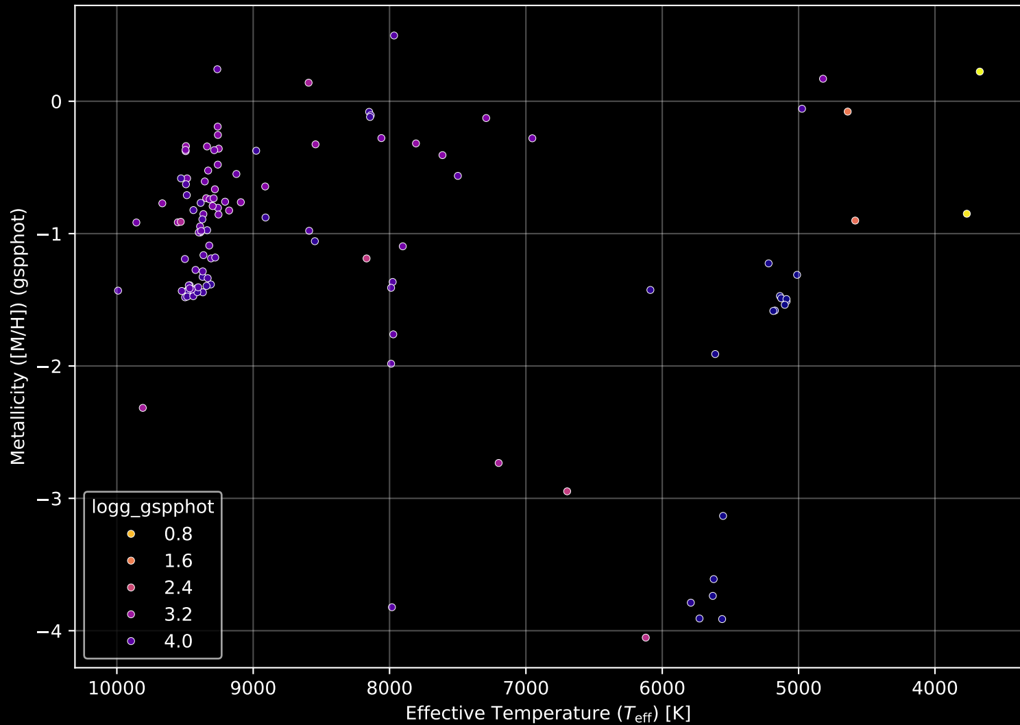
Gaia Cluster: [Ruprecht_83] Stellar Population Parameters (n= 120)
