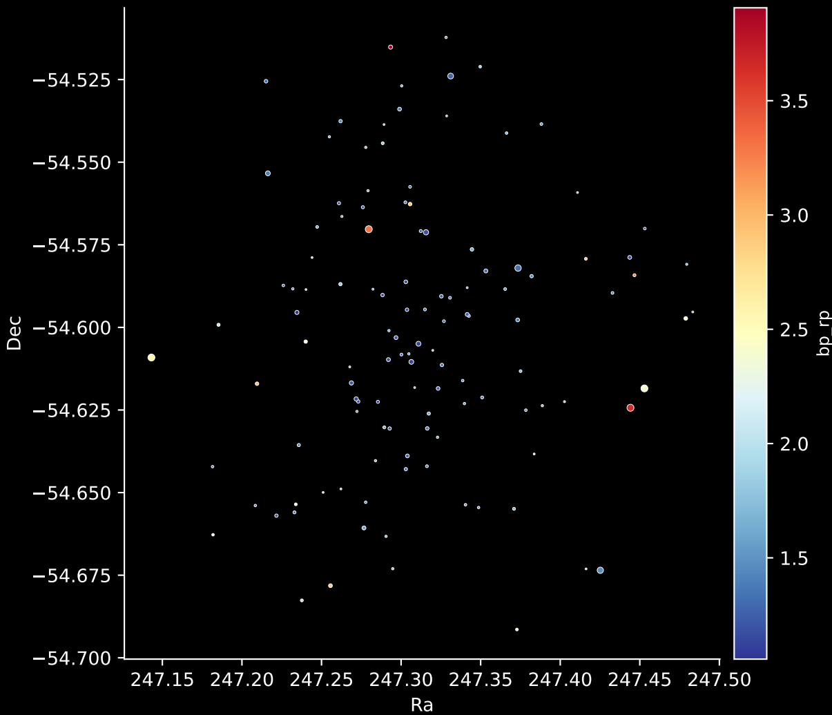
Gaia Cluster: [Ruprecht_83] Stars: 120
