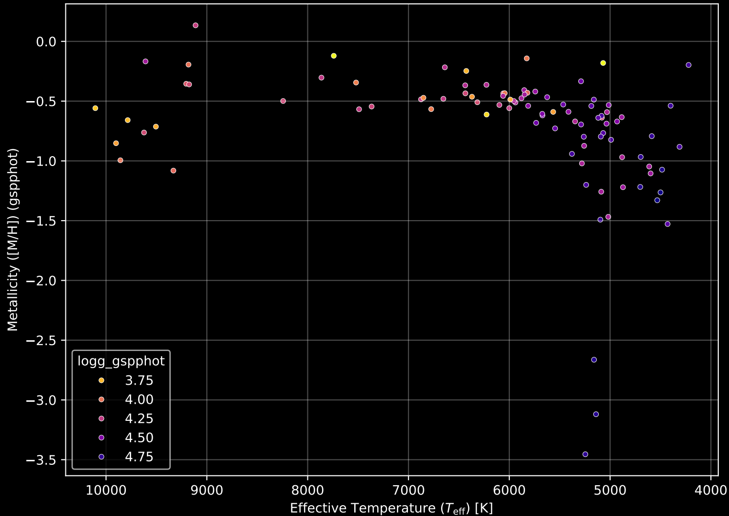
Gaia Cluster: [Ruprecht_84] Stellar Population Parameters (n= 95)
