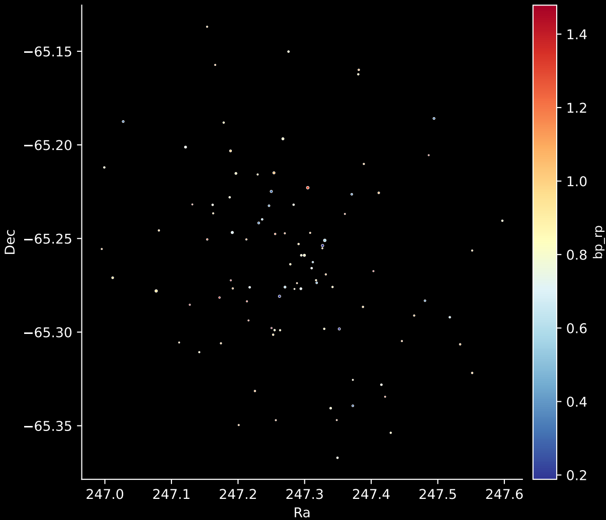
Gaia Cluster: [Ruprecht_84] Stars: 95
