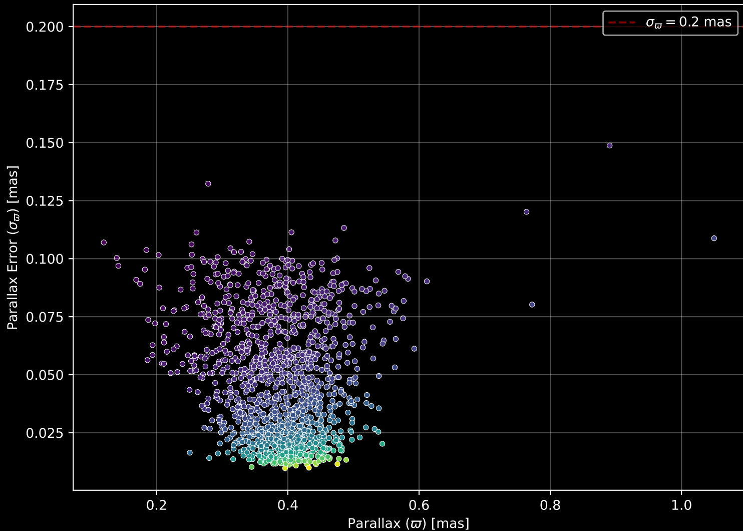
Gaia Cluster: [Ruprecht_94] Parallax Quality (n= 1331)
