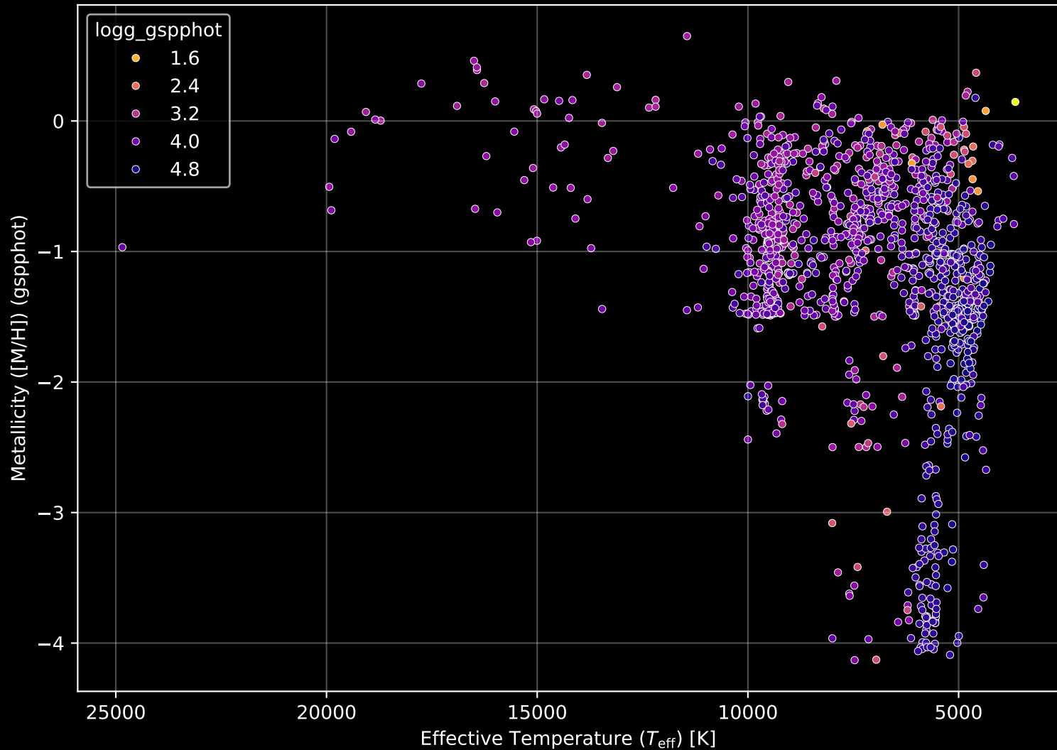
Gaia Cluster: [Ruprecht_94] Stellar Population Parameters (n= 1331)
