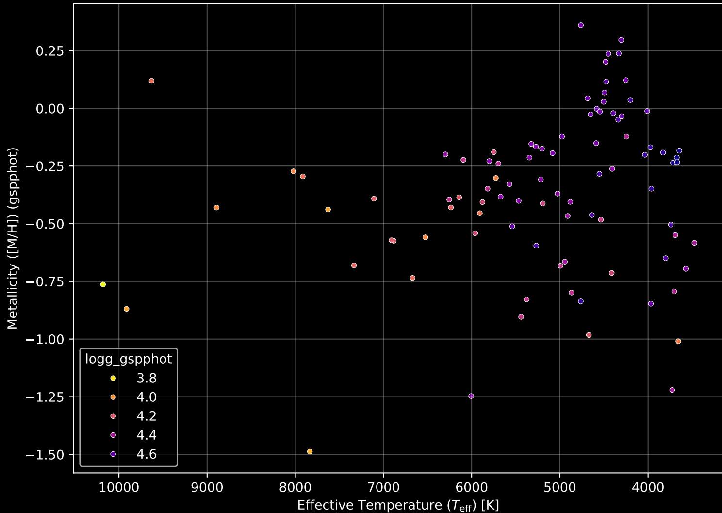
Gaia Cluster: [Ruprecht_98] Stellar Population Parameters (n= 93)
