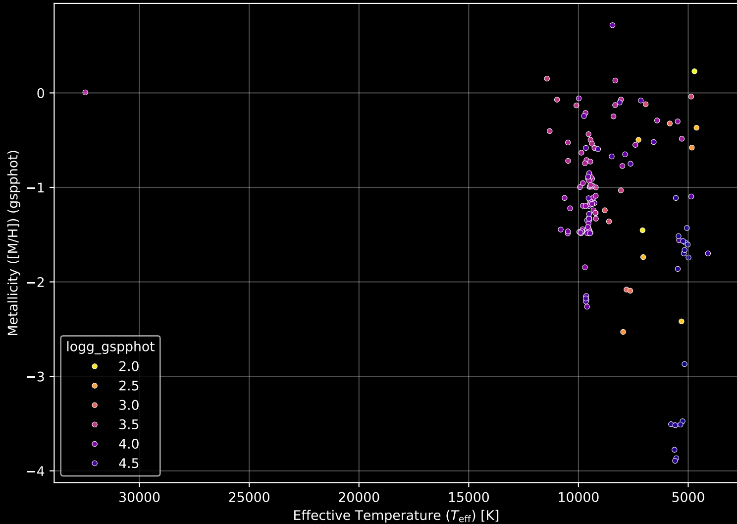
Gaia Cluster: [SAI_113] Stellar Population Parameters (n= 142)
