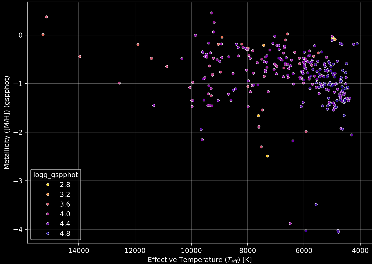
Gaia Cluster: [SAI_118] Stellar Population Parameters (n= 293)
