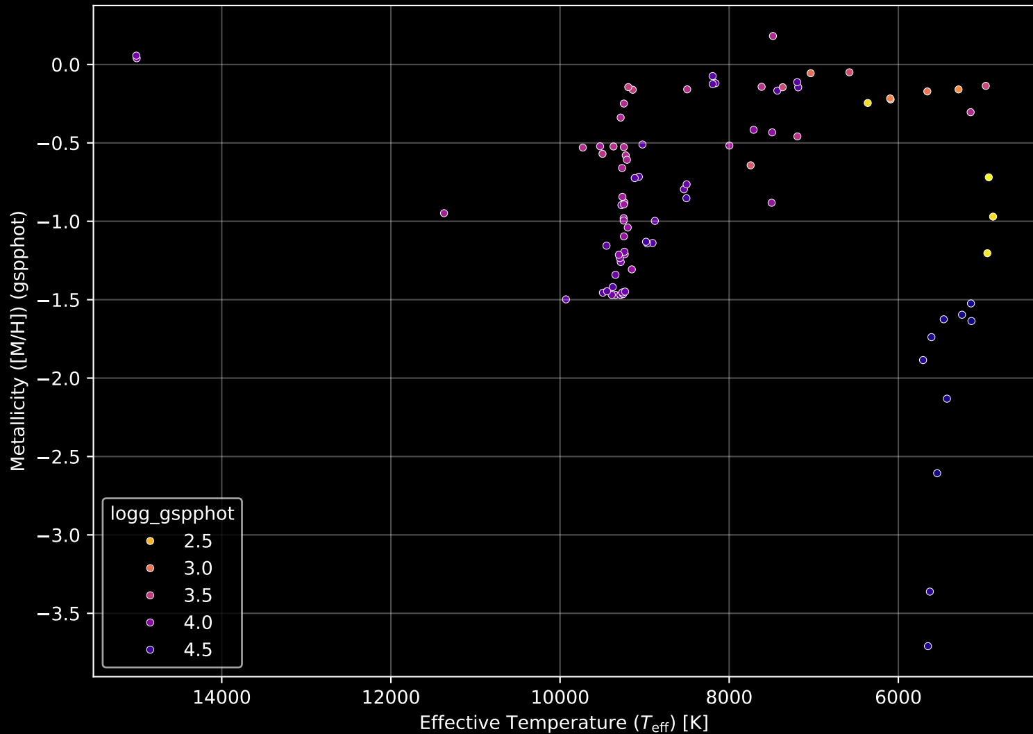
Gaia Cluster: [SAI_14] Stellar Population Parameters (n= 90)
