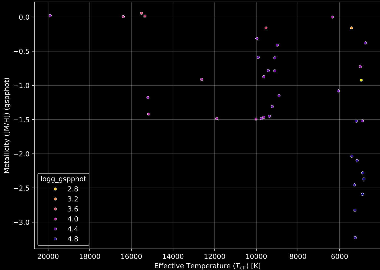
Gaia Cluster: [SAI_47] Stellar Population Parameters (n= 38)
