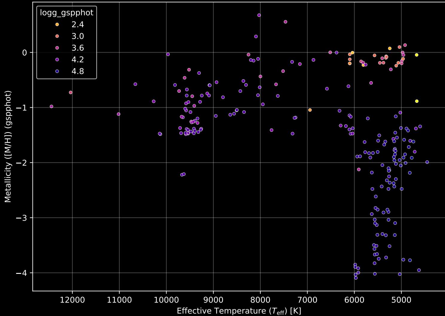
Gaia Cluster: [SAI_94] Stellar Population Parameters (n= 225)
