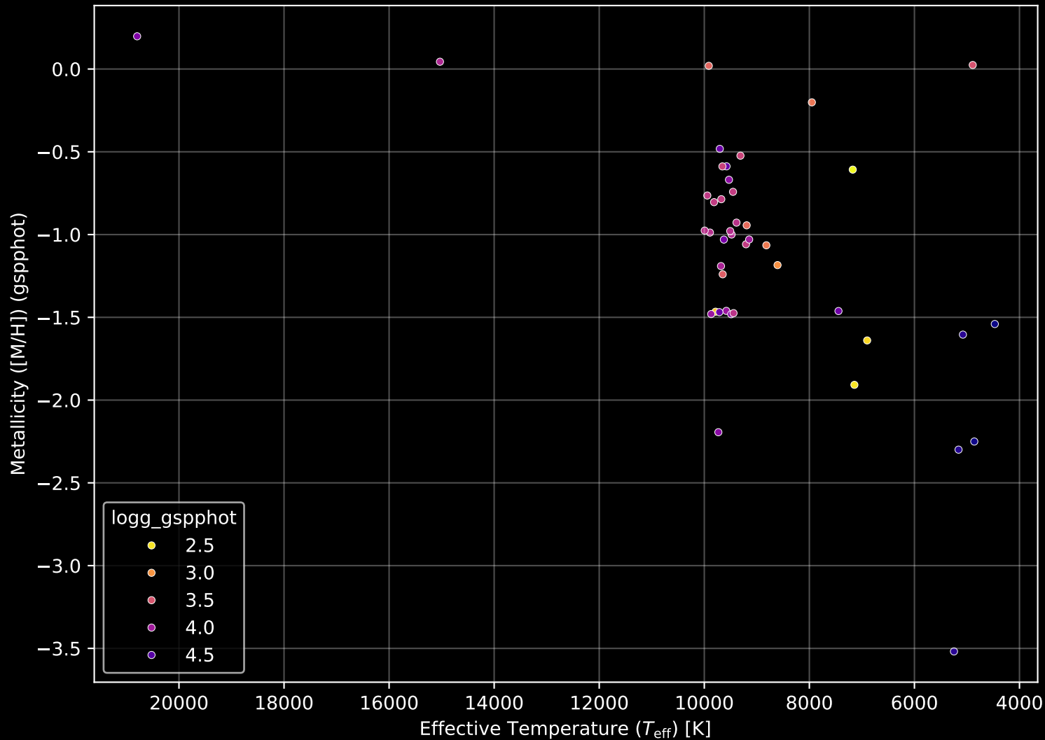
Gaia Cluster: [Shorlin_1] Stellar Population Parameters (n= 43)
