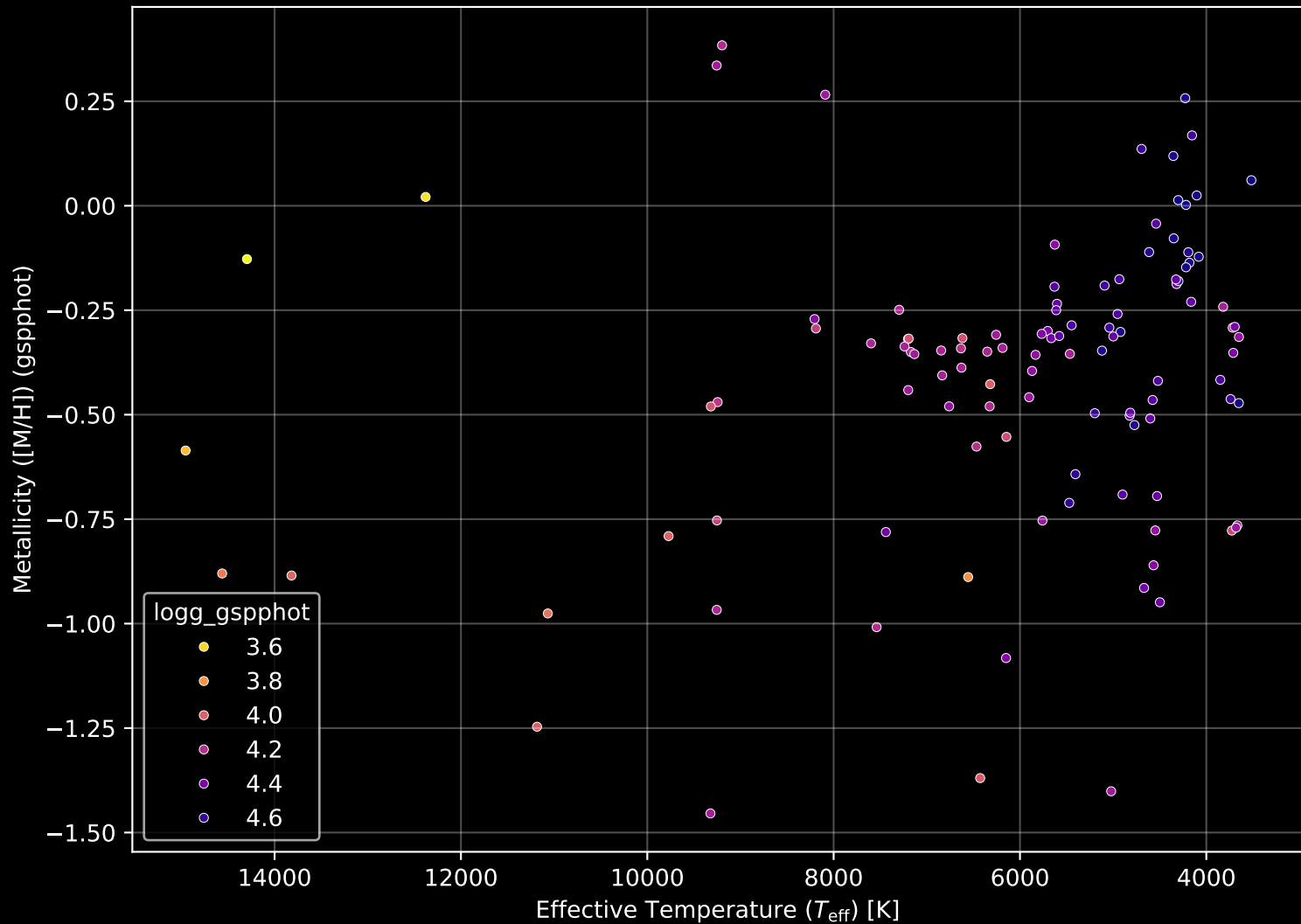
Gaia Cluster: [Stock_23] Stellar Population Parameters (n= 111)
