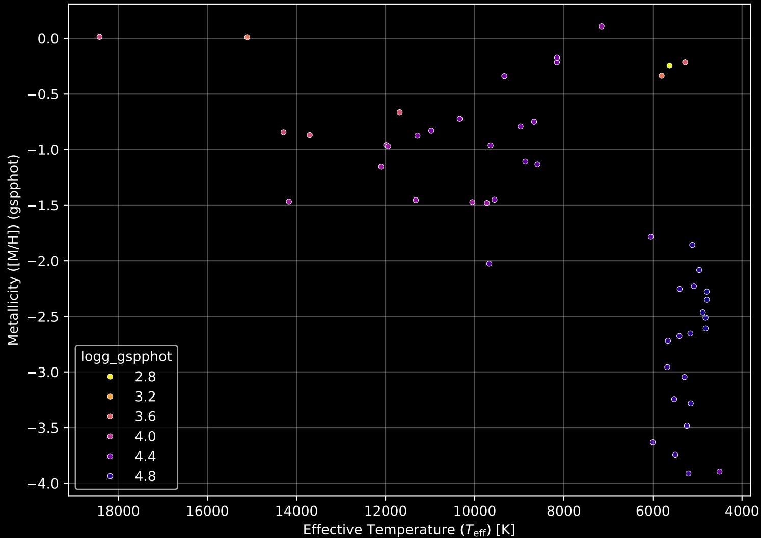
Gaia Cluster: [Deutsch_1] Stellar Population Parameters (n= 51)
