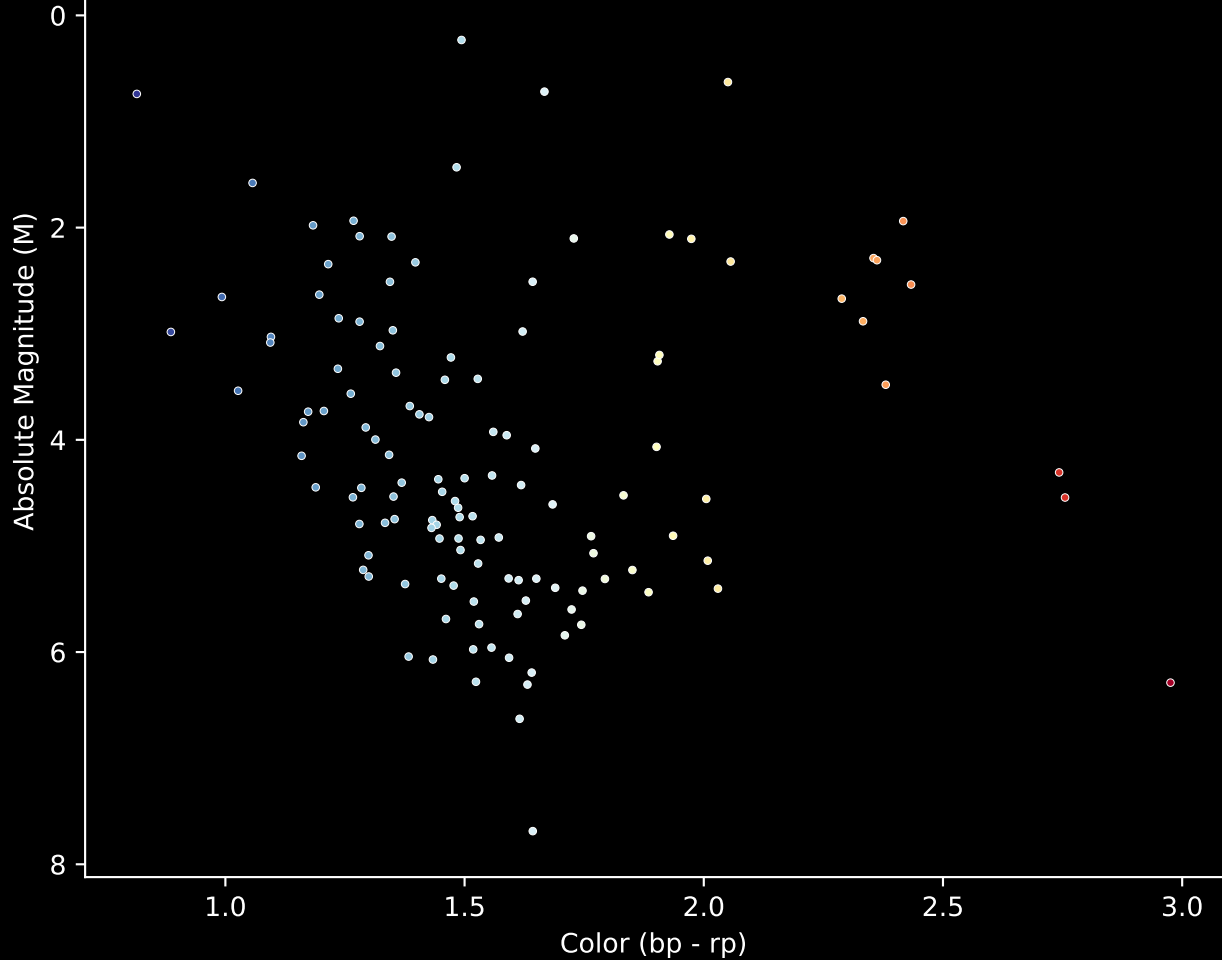
Gaia Cluster: [Deutsch_10] Stars (n= 128) Hertzsprung-Russel Diagram
