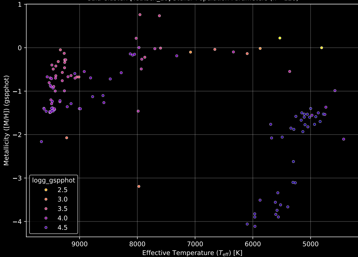
Gaia Cluster: [Deutsch_10] Stellar Population Parameters (n= 128)
