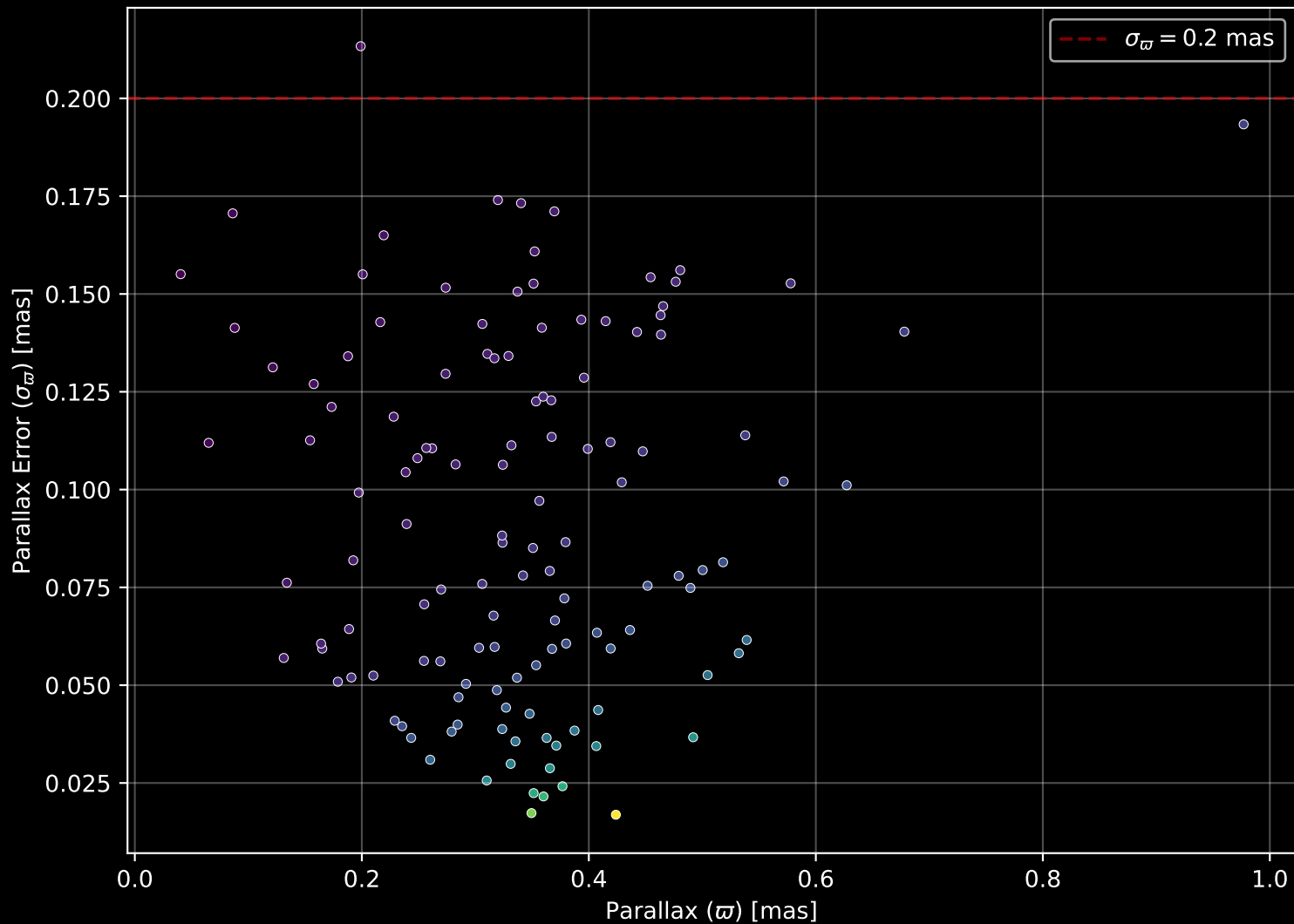
Gaia Cluster: [Deutsch_10] Parallax Quality (n= 128)
