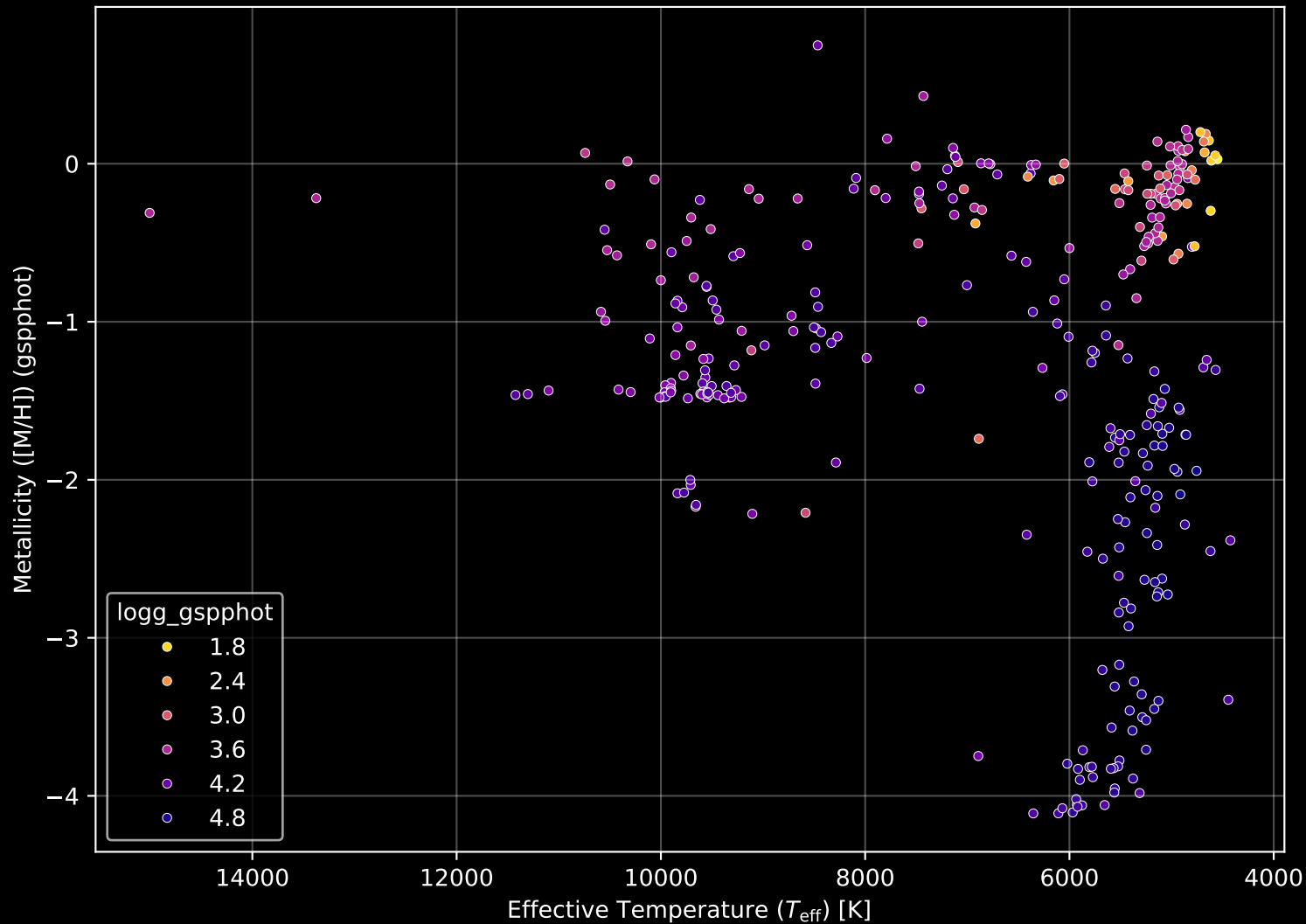
Gaia Cluster: [Teutsch_106] Stellar Population Parameters (n= 332)
