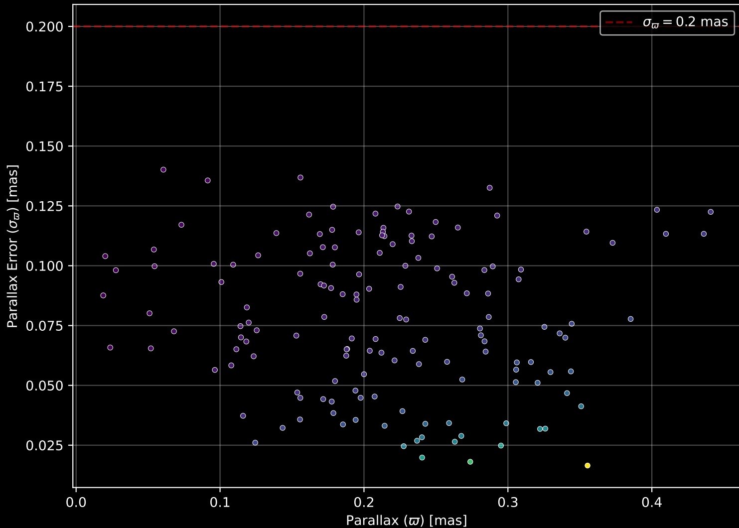
Gaia Cluster: [Deutsch_11] Parallax Quality (n= 148)
