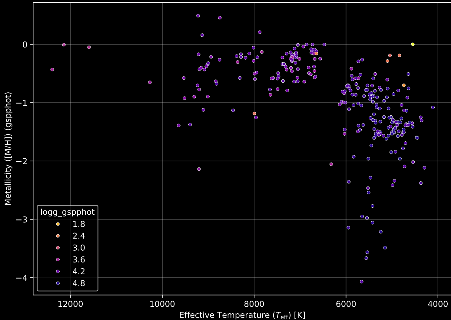
Gaia Cluster: [Teutsch_126] Stellar Population Parameters (n= 268)
