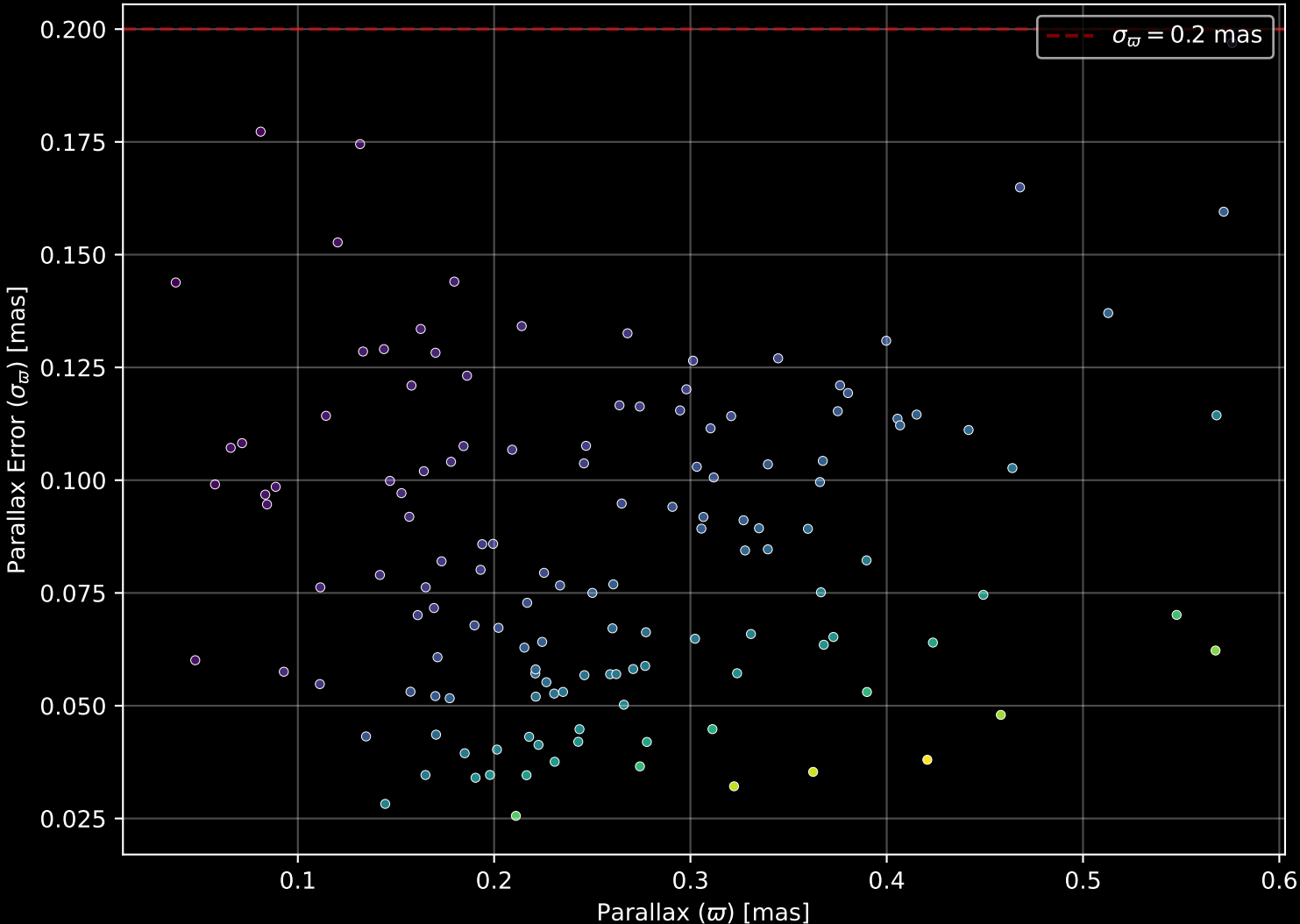
Gaia Cluster: [Deutsch 145] Parallax Quality (n= 138)
