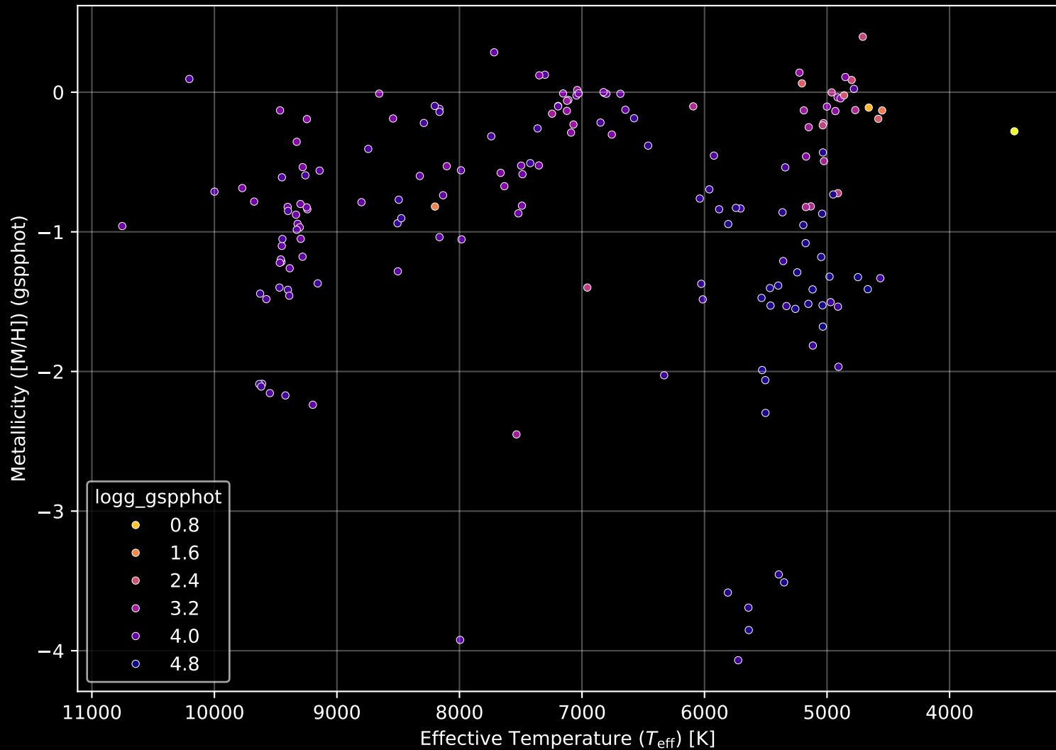
Gaia Cluster: [Teutsch_156] Stellar Population Parameters (n= 171)
