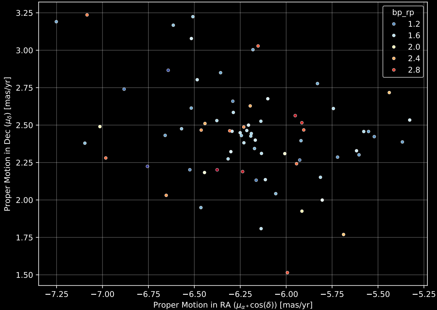
Gaia Cluster: [Deutsch_31] Proper Motion Diagram (n= 74)
