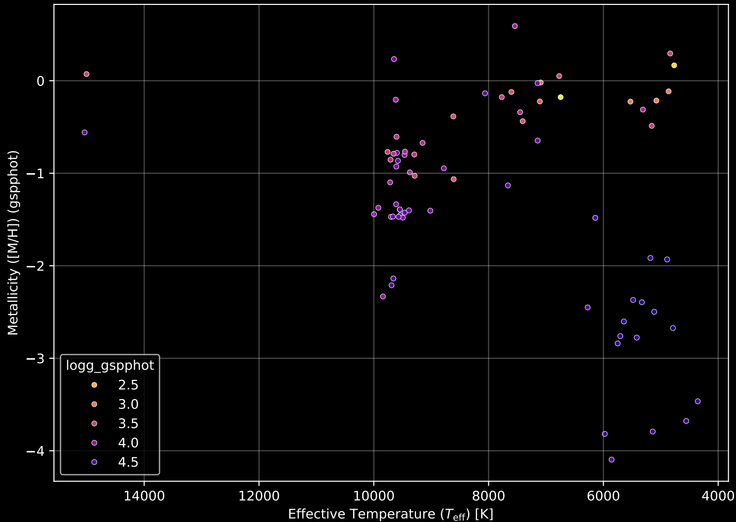
Gaia Cluster: [Teutsch_31] Stellar Population Parameters (n= 74)
