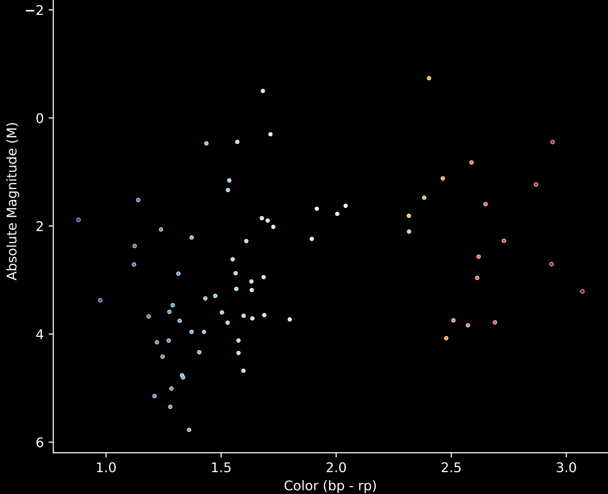
Gaia Cluster: [Teutsch_31] Stars (n= 74) Hertzsprung-Russel Diagram
