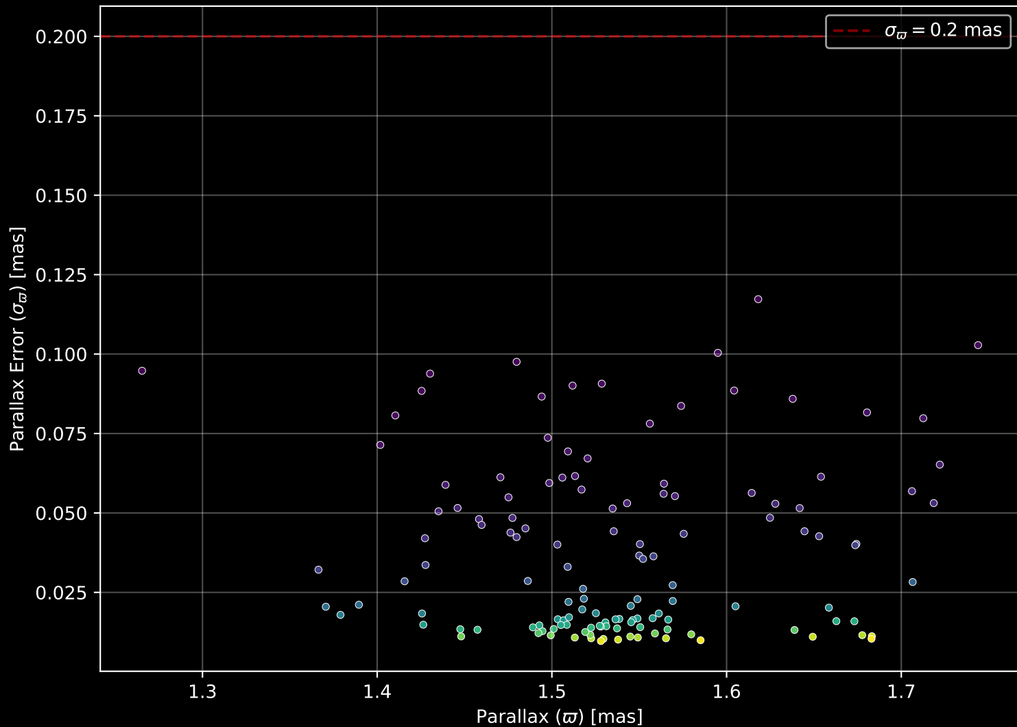
Gaia Cluster: [Deutsch_38] Parallax Quality (n= 133)
