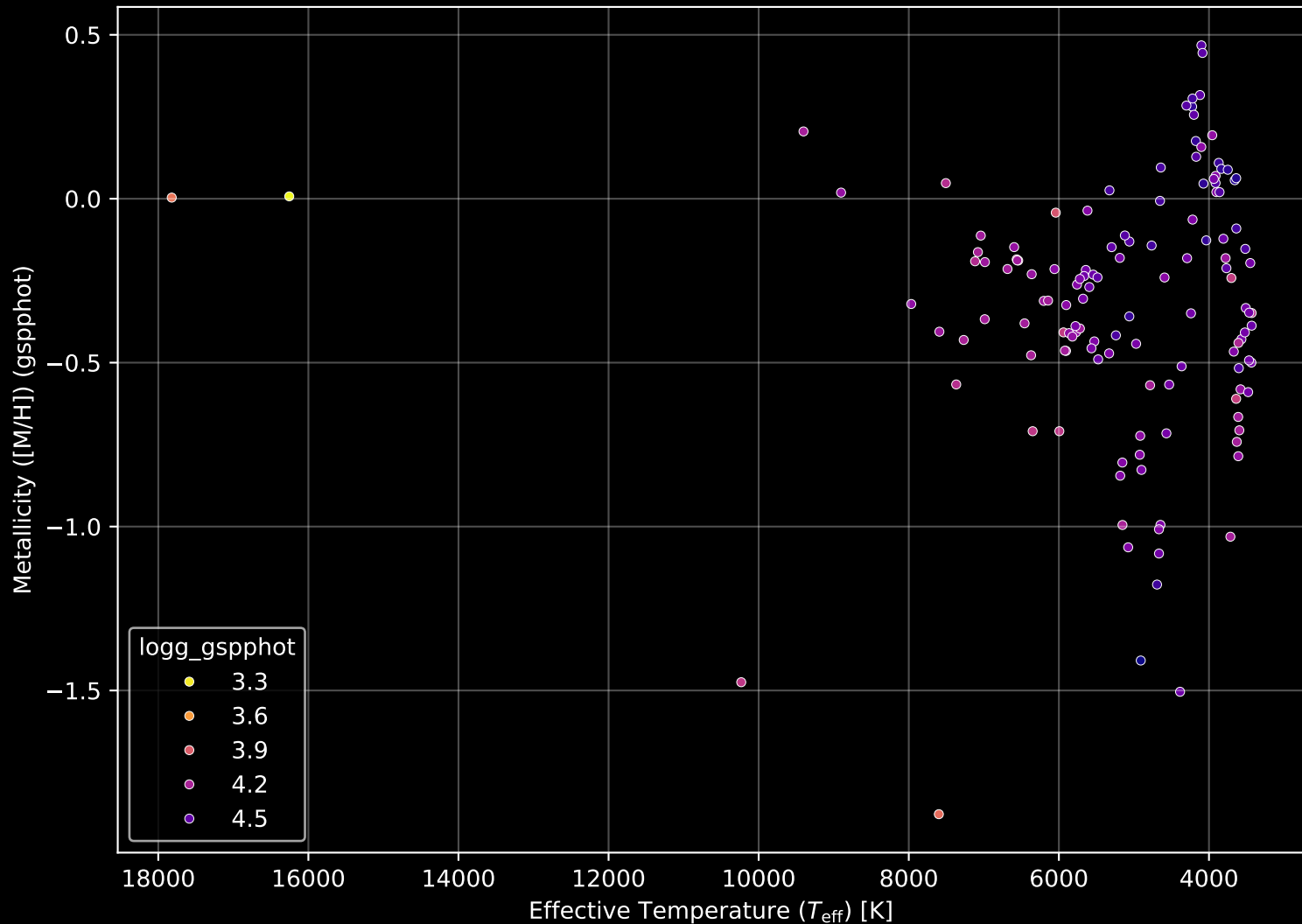
Gaia Cluster: [Teutsch_38] Stellar Population Parameters (n= 133)
