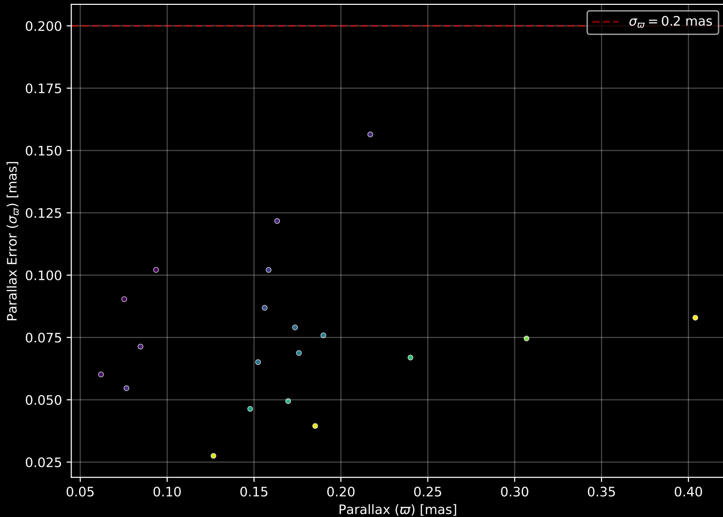
Gaia Cluster: [Deutsch_42] Parallax Quality (n= 20)
