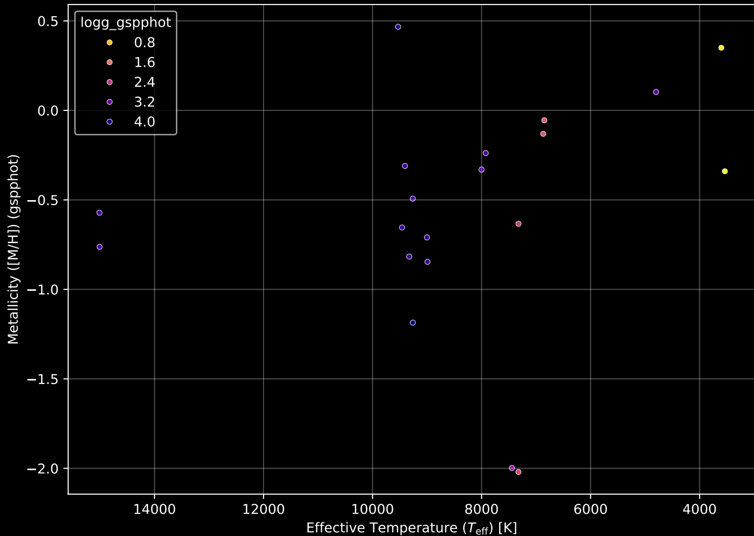
Gaia Cluster: [Teutsch_42] Stellar Population Parameters (n= 20)
