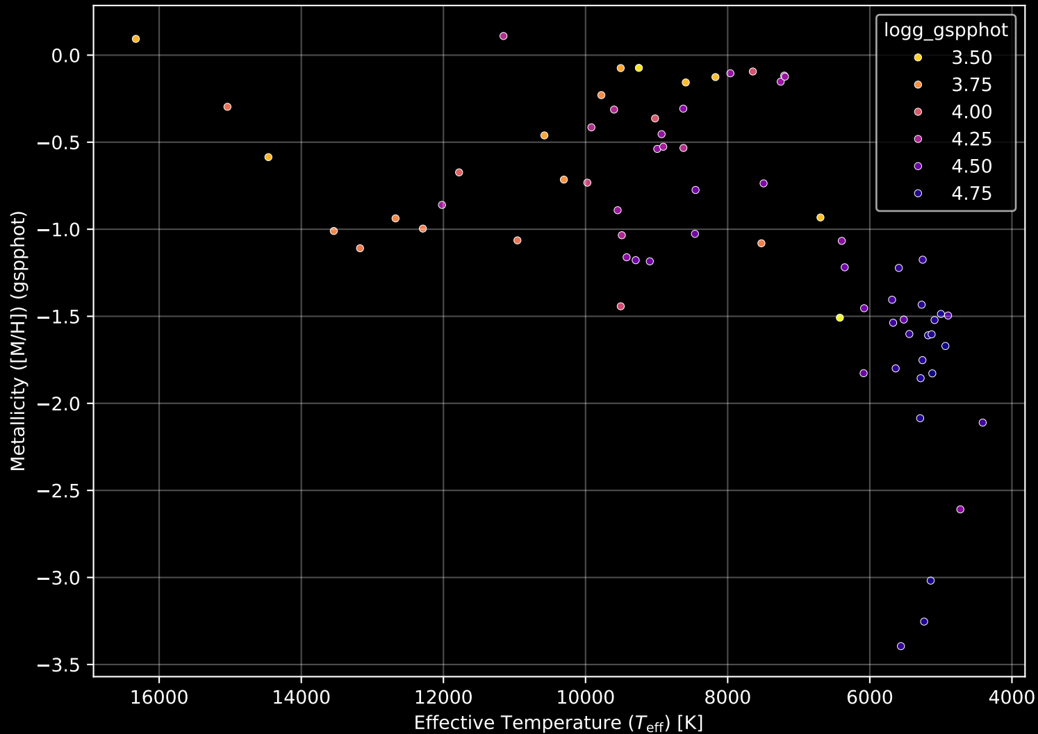
Gaia Cluster: [Teutsch_61] Stellar Population Parameters (n= 71)
