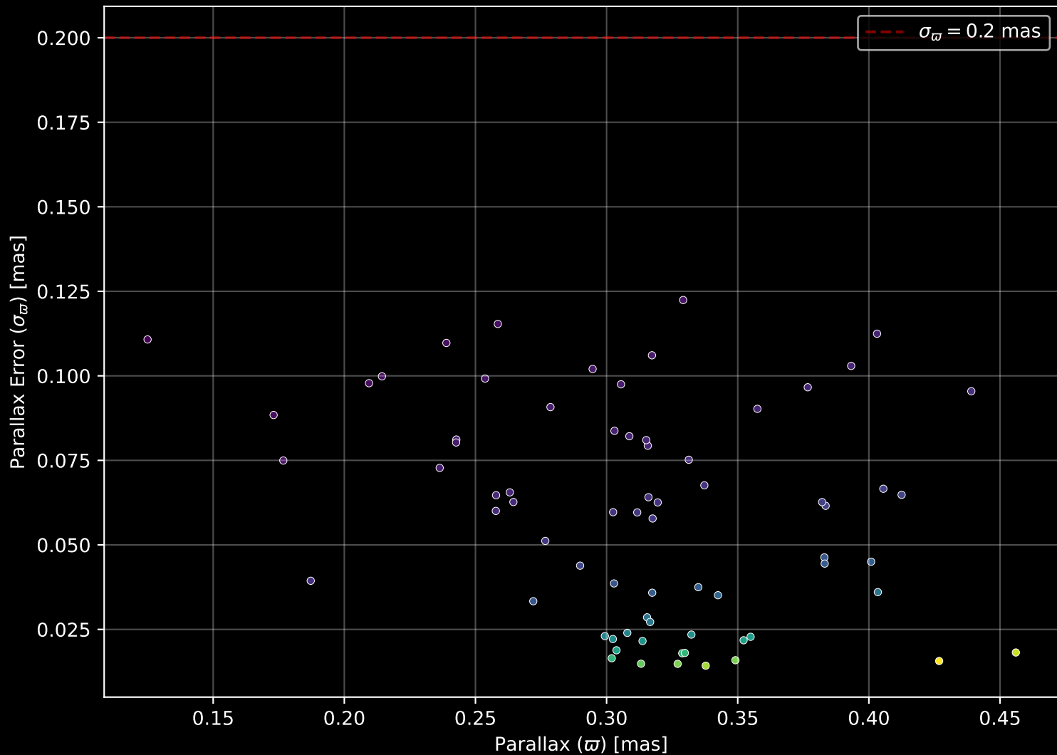
Gaia Cluster: [Deutsch_61] Parallax Quality (n= 71)
