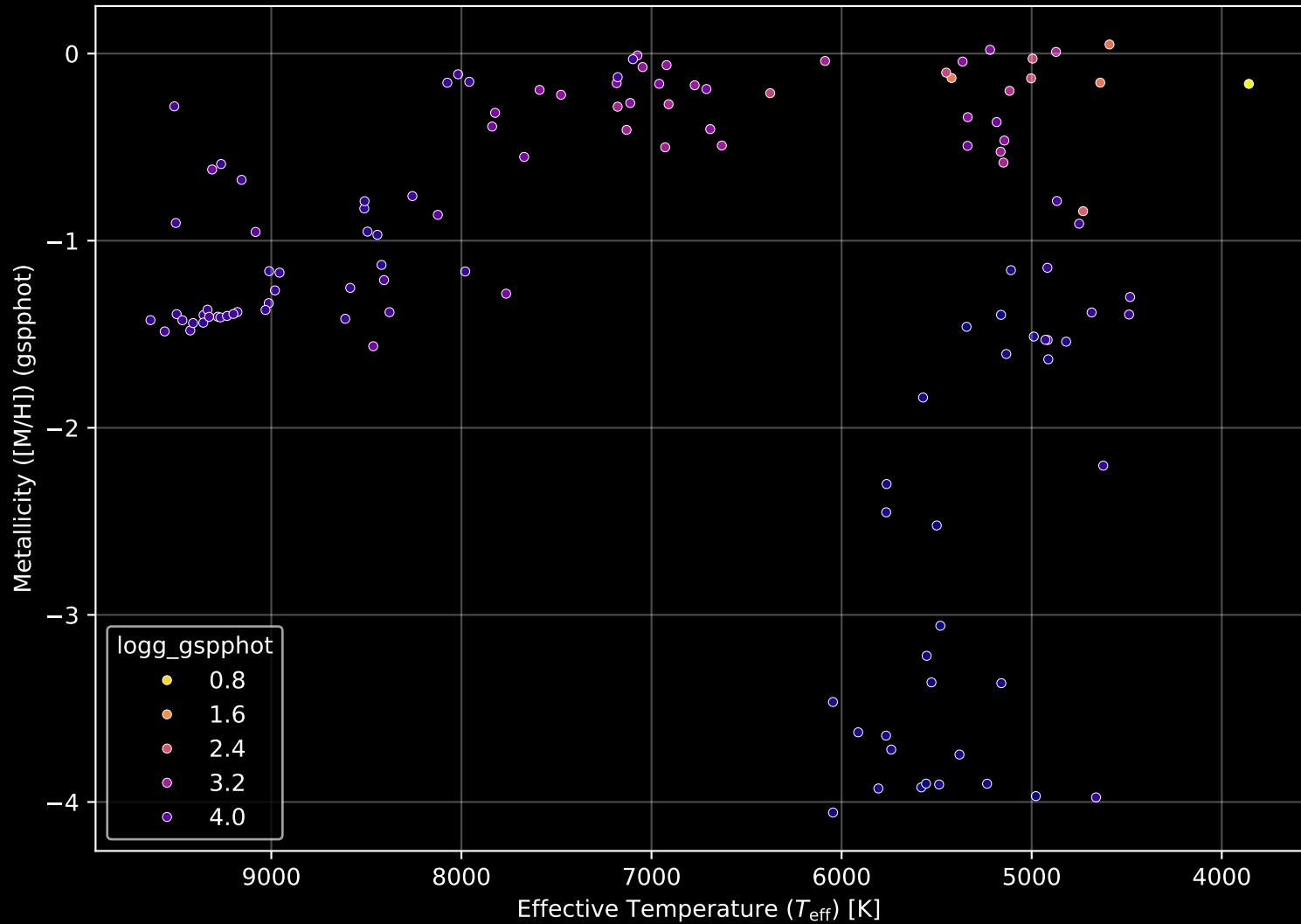
Gaia Cluster: [Deutsch_74] Stellar Population Parameters (n= 121)
