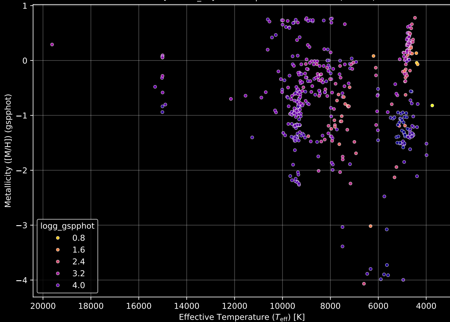
Gaia Cluster: [Teutsch_85] Stellar Population Parameters (n= 475)
