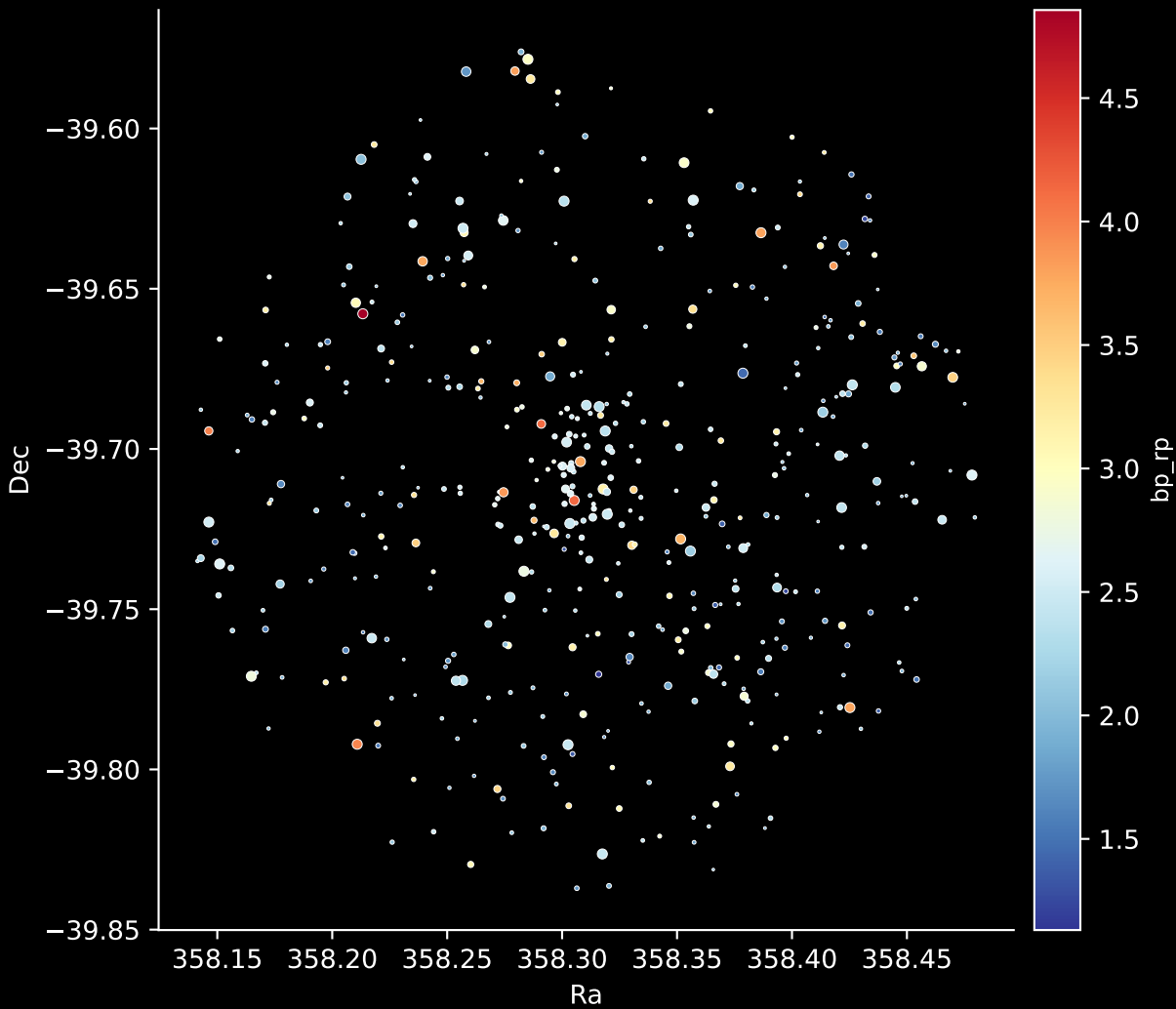
Gaia Cluster: [Deutsch_85] Stars: 475
