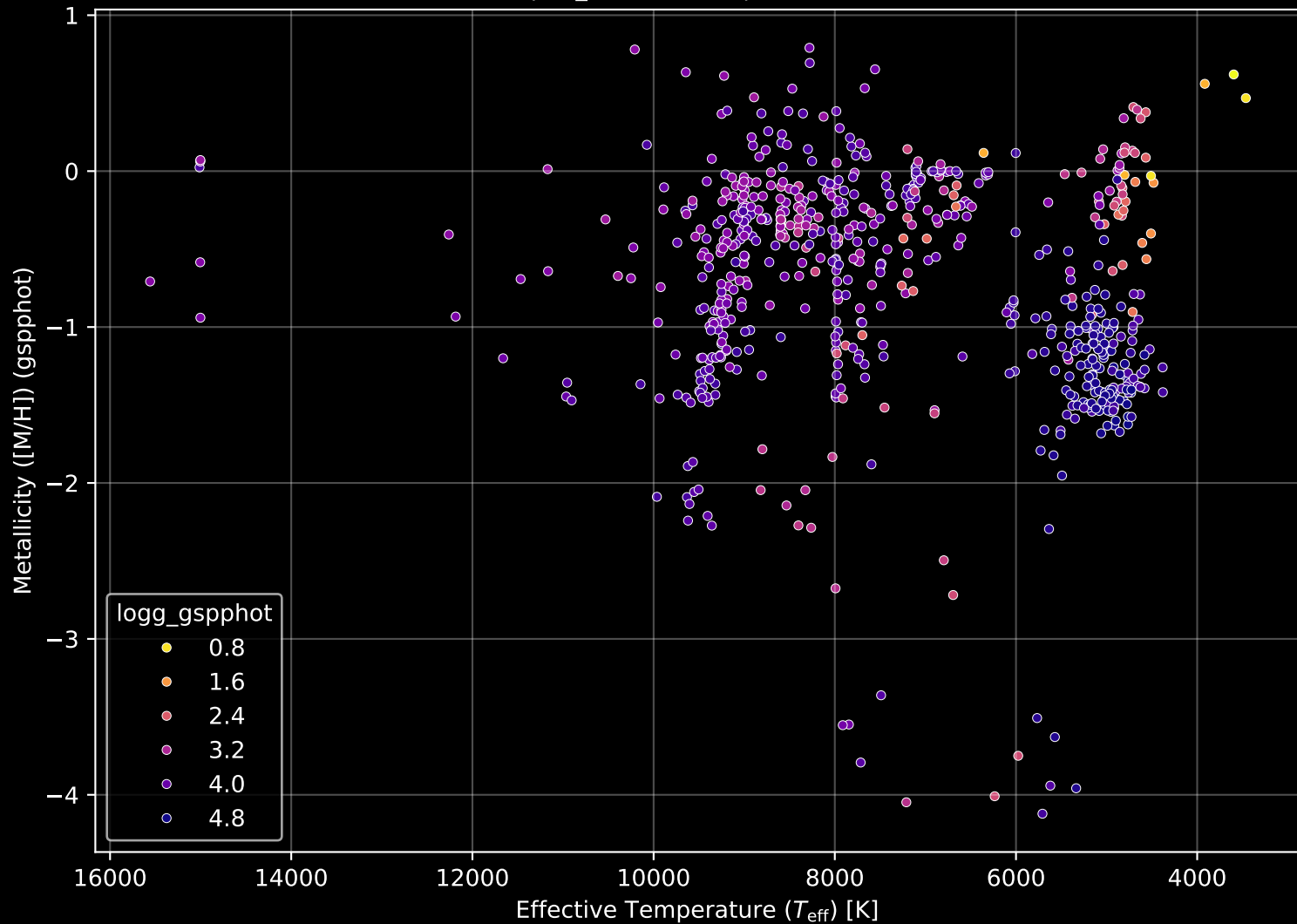
Gaia Cluster: [Trumpler_22] Stellar Population Parameters (n= 692)
