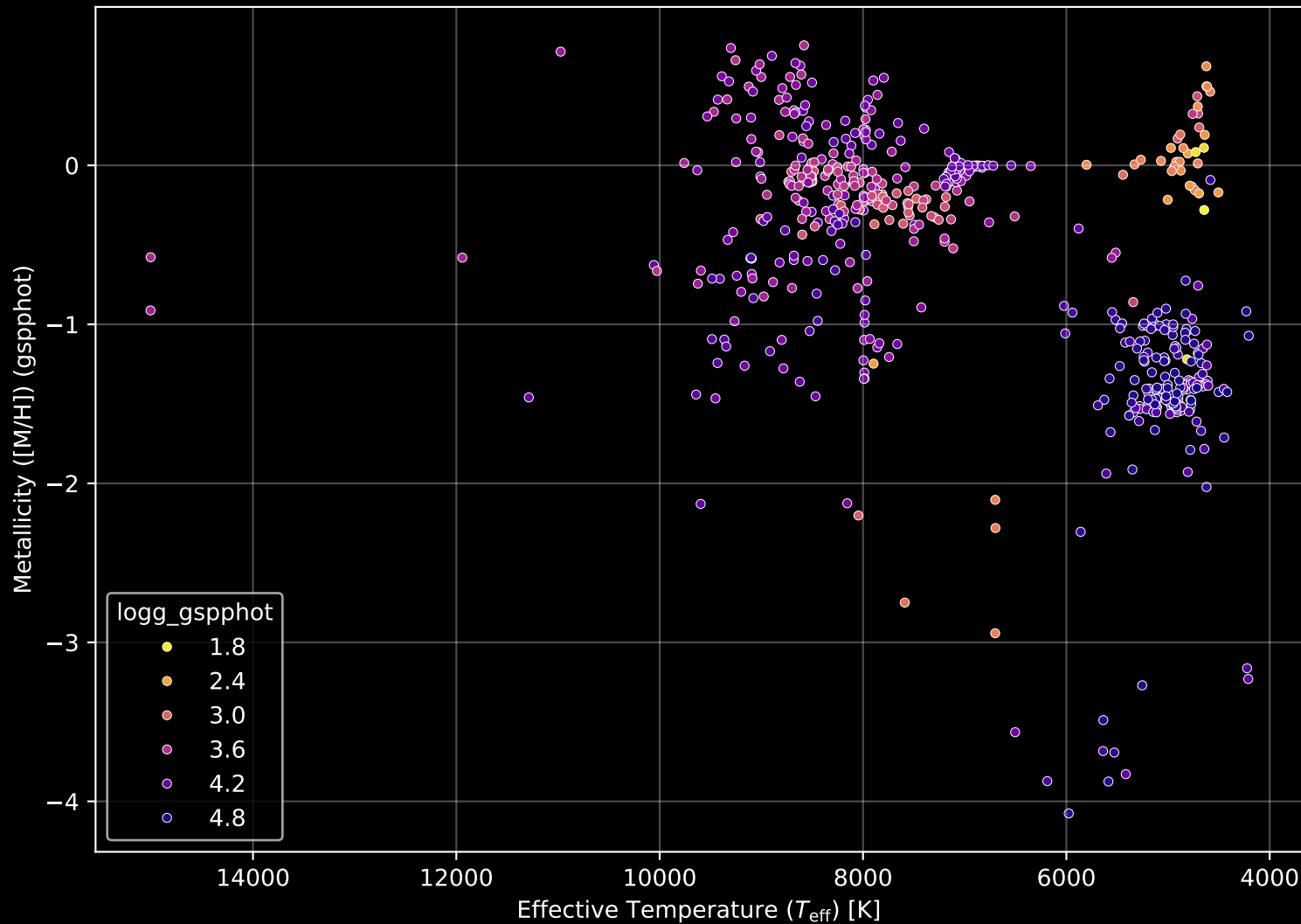
Gaia Cluster: [Trumpler_23] Stellar Population Parameters (n= 554)
