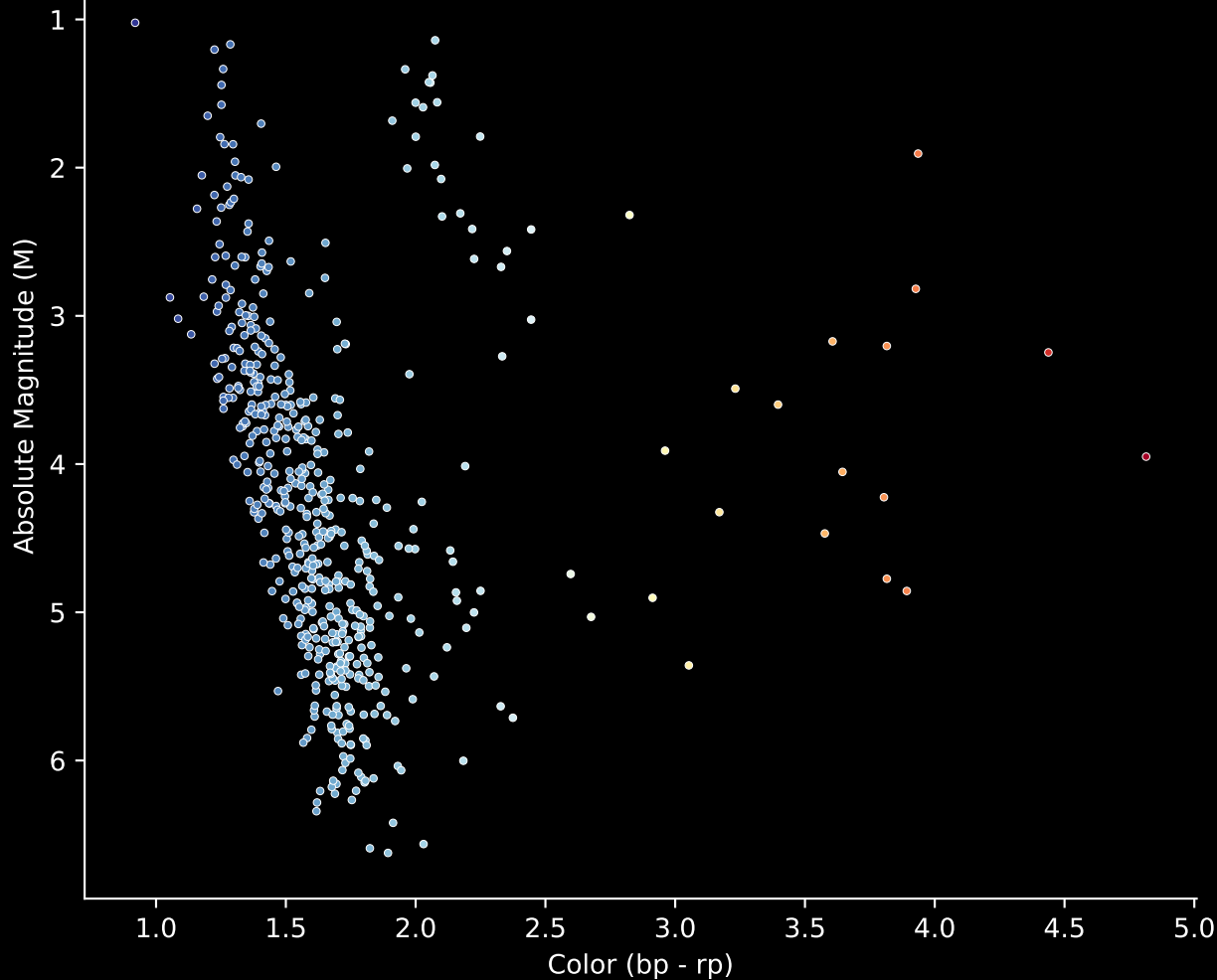
Gaia Cluster: [Trumpler_23] Stars (n= 554) Hertzsprung-Russel Diagram
