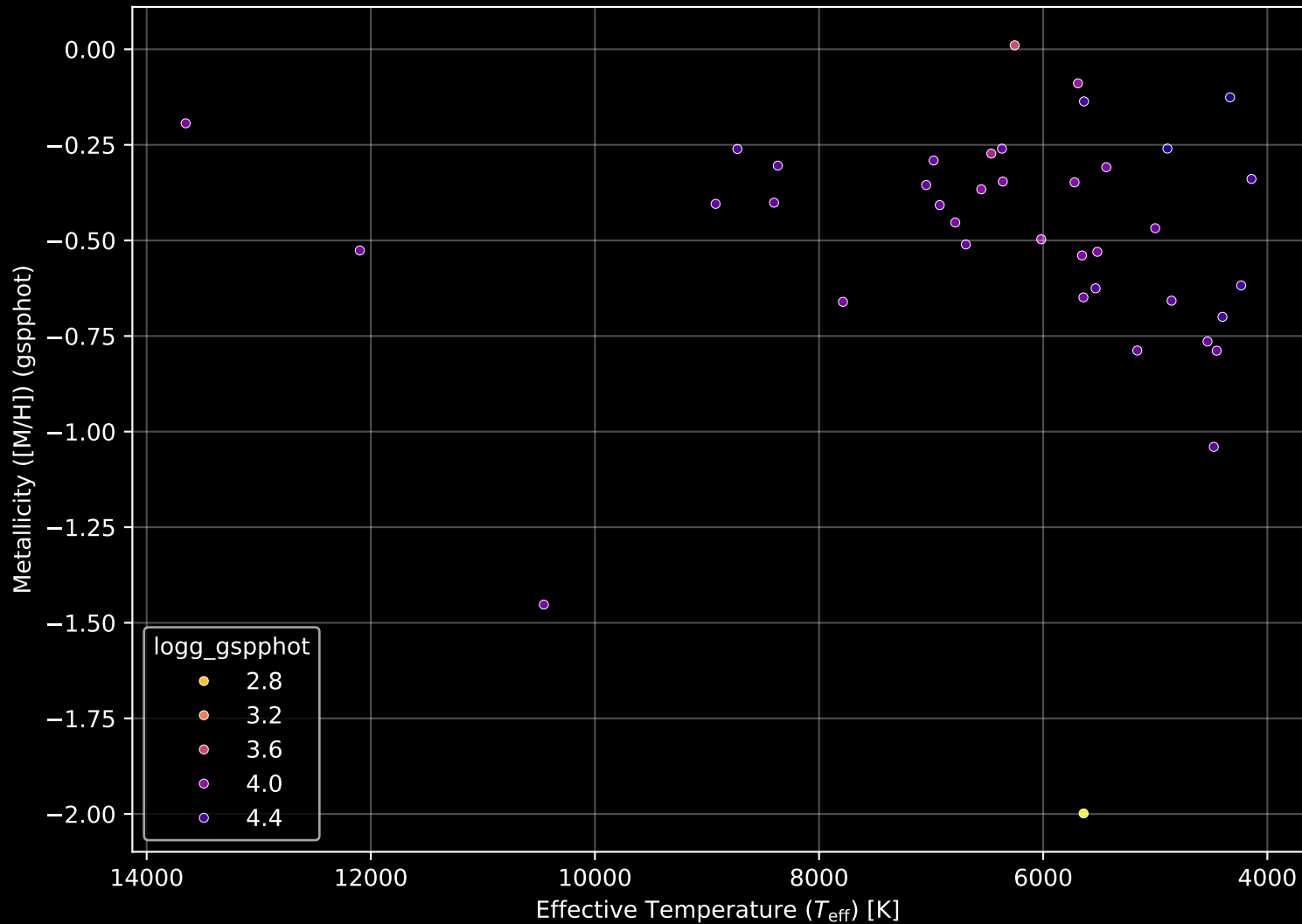
Gaia Cluster: [UBC_10a] Stellar Population Parameters (n= 39)
