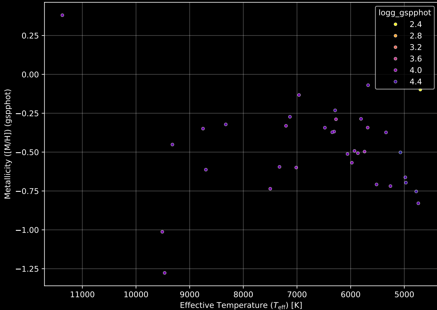
Gaia Cluster: [UBC_10b] Stellar Population Parameters (n= 35)
