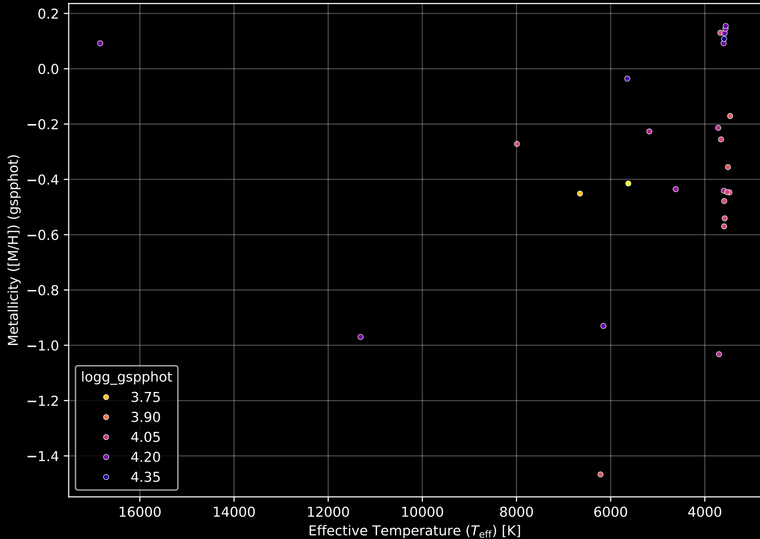
Gaia Cluster: [UBC_19] Stellar Population Parameters (n= 27)
