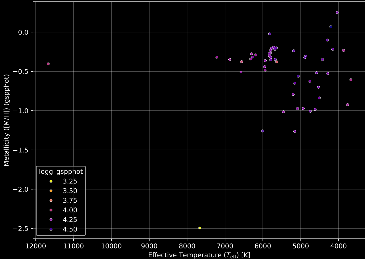
Gaia Cluster: [UBC_26] Stellar Population Parameters (n= 52)
