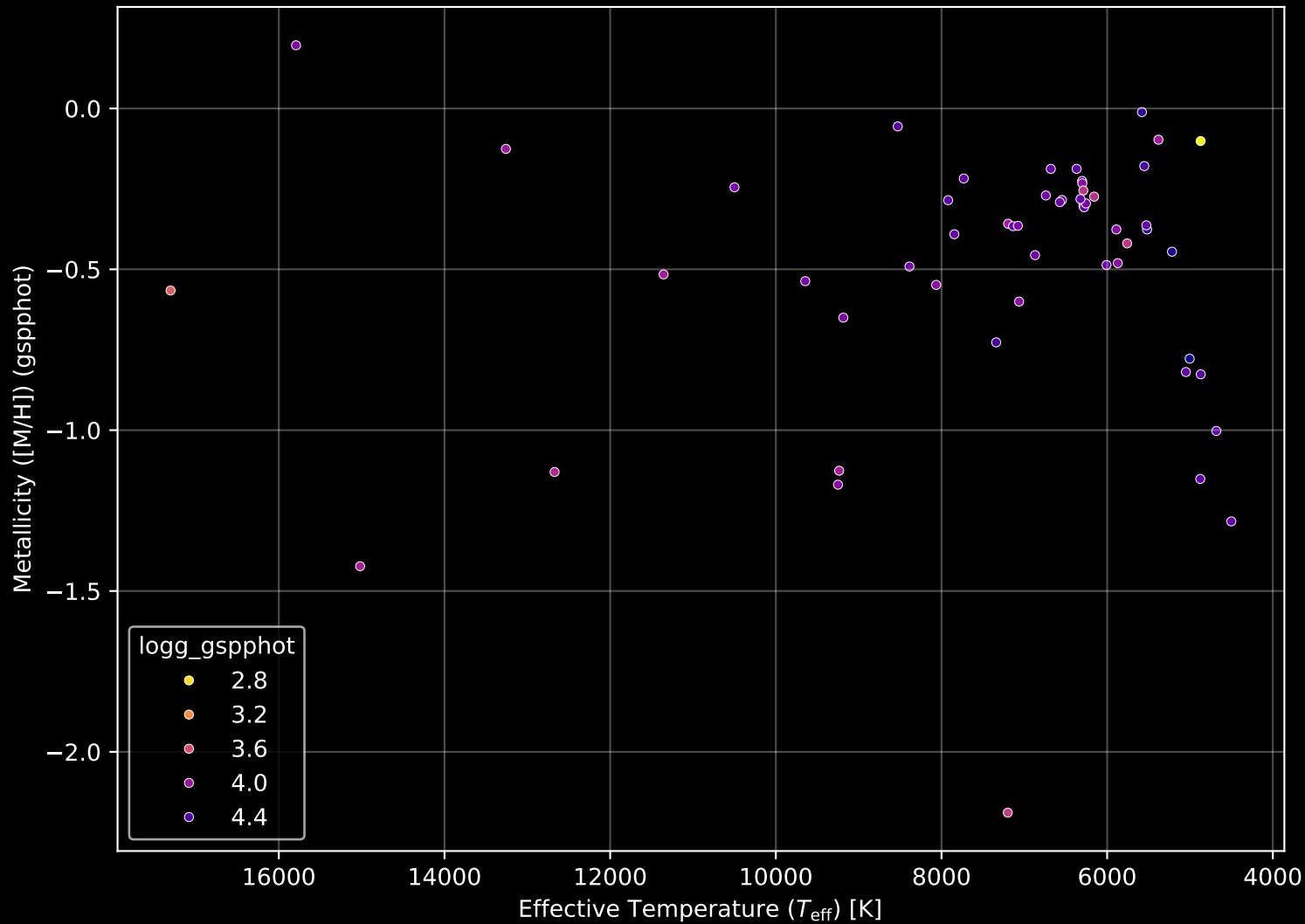
Gaia Cluster: [UBC_55] Stellar Population Parameters (n= 54)
