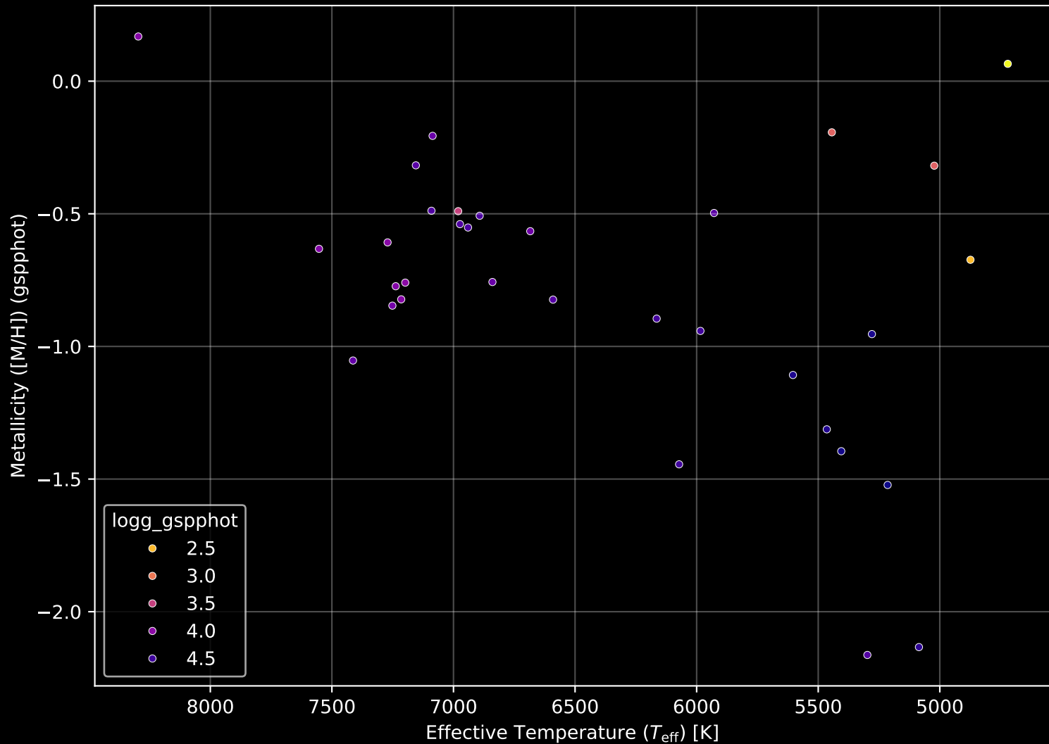
Gaia Cluster: [UBC_57] Stellar Population Parameters (n= 33)
