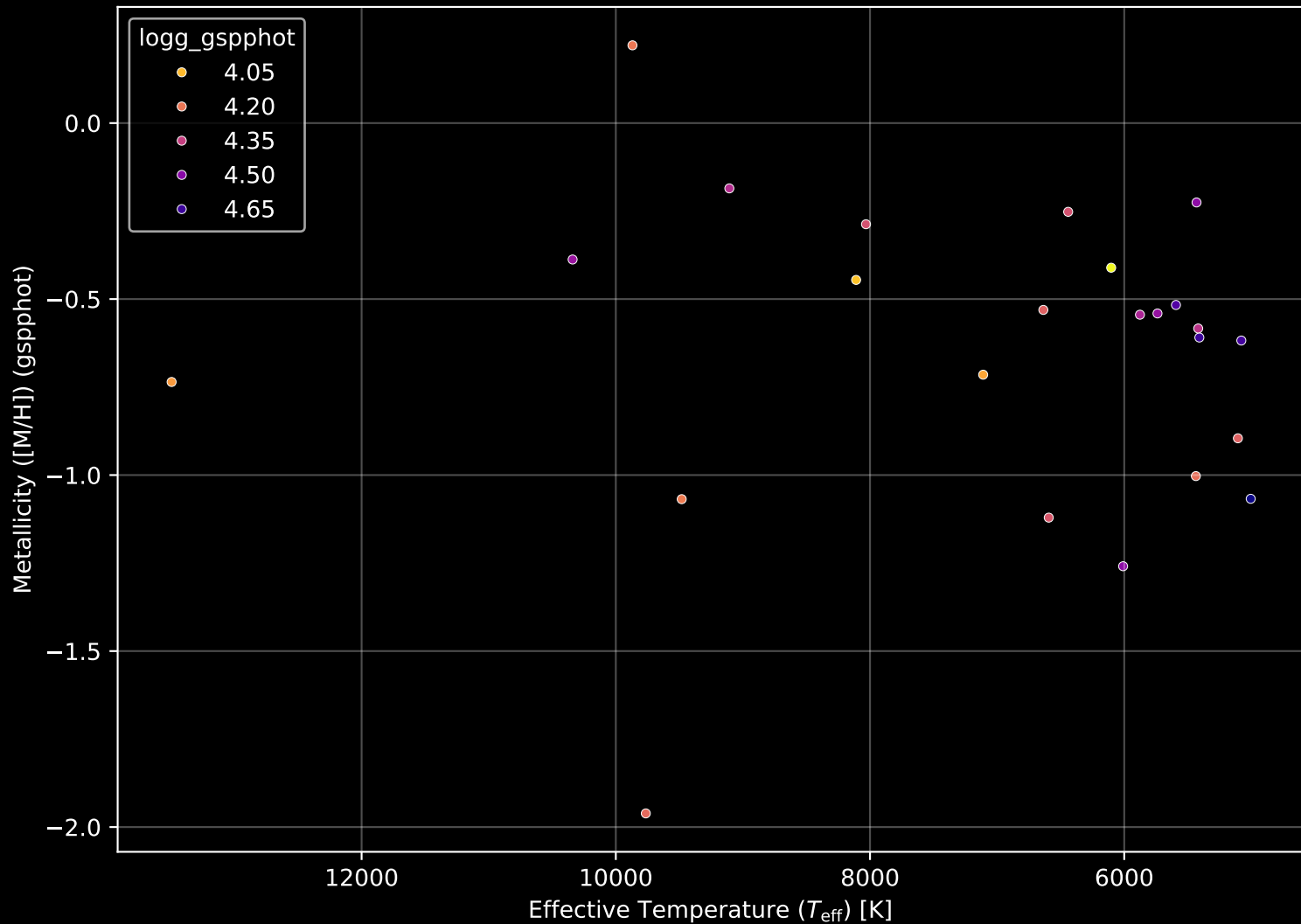
Gaia Cluster: [UBC_63] Stellar Population Parameters (n= 24)
