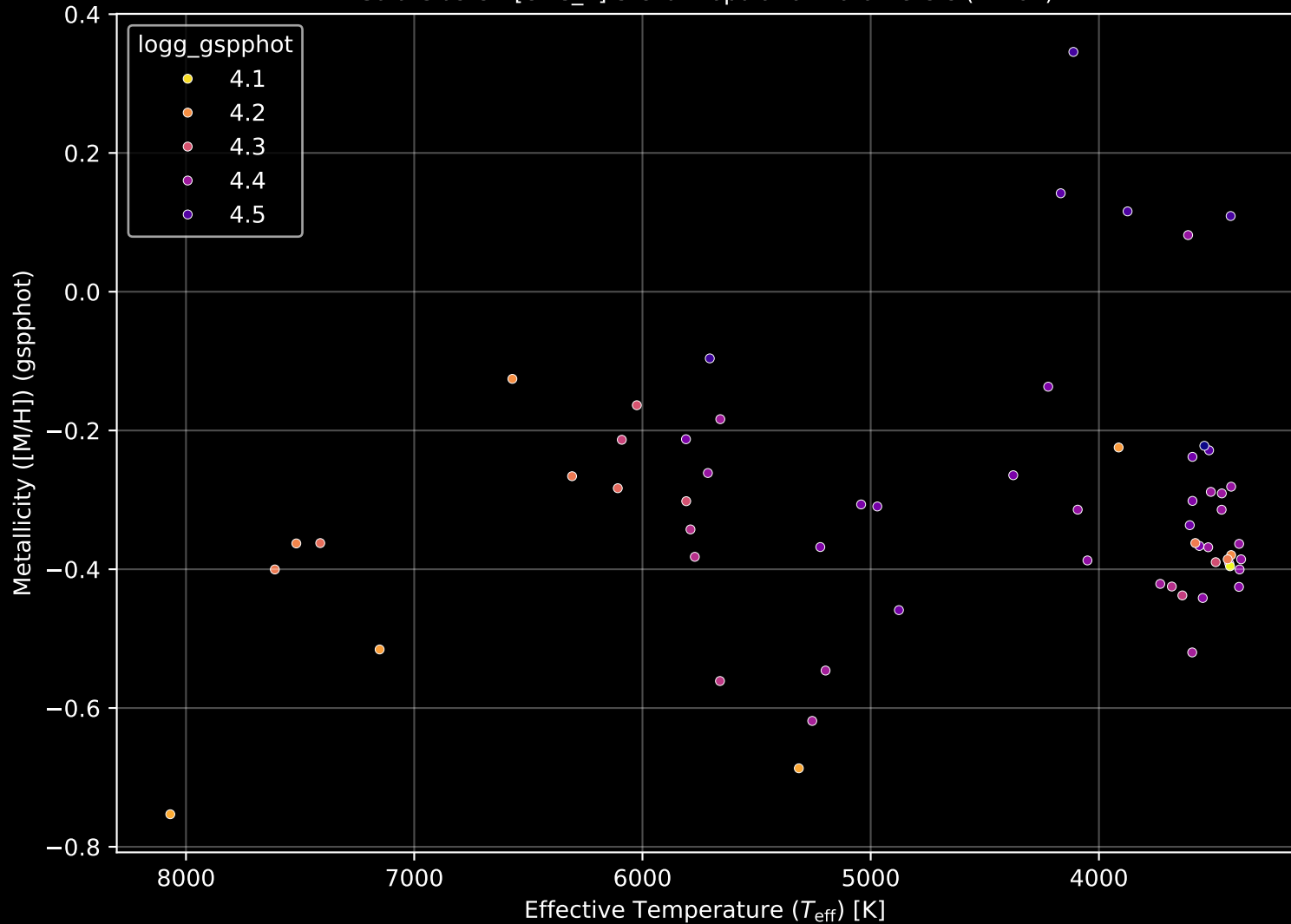
Gaia Cluster: [UBC_7] Stellar Population Parameters (n= 61)
