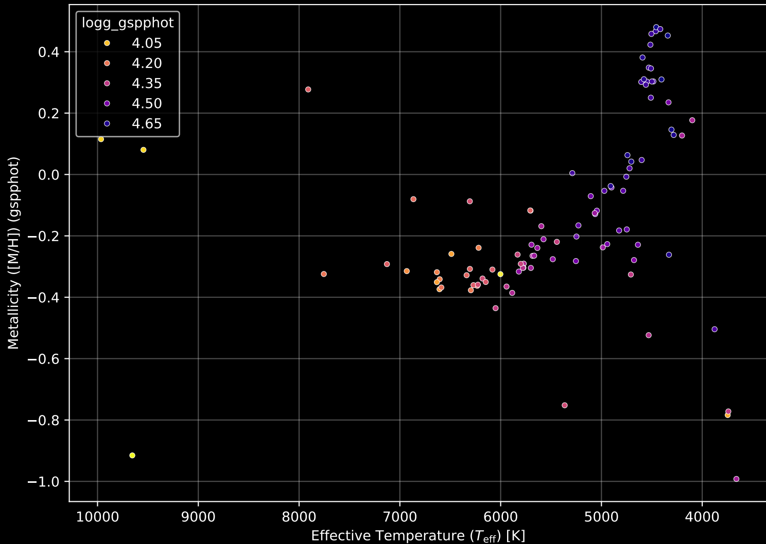
Gaia Cluster: [UBC_8] Stellar Population Parameters (n= 99)
