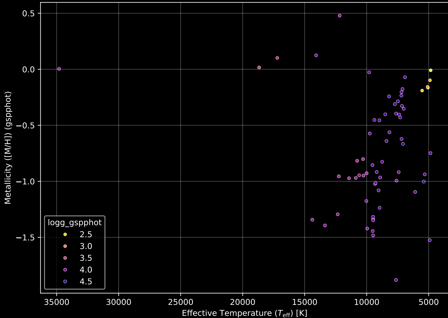
Gaia Cluster: [UBC_86] Stellar Population Parameters (n= 65)
