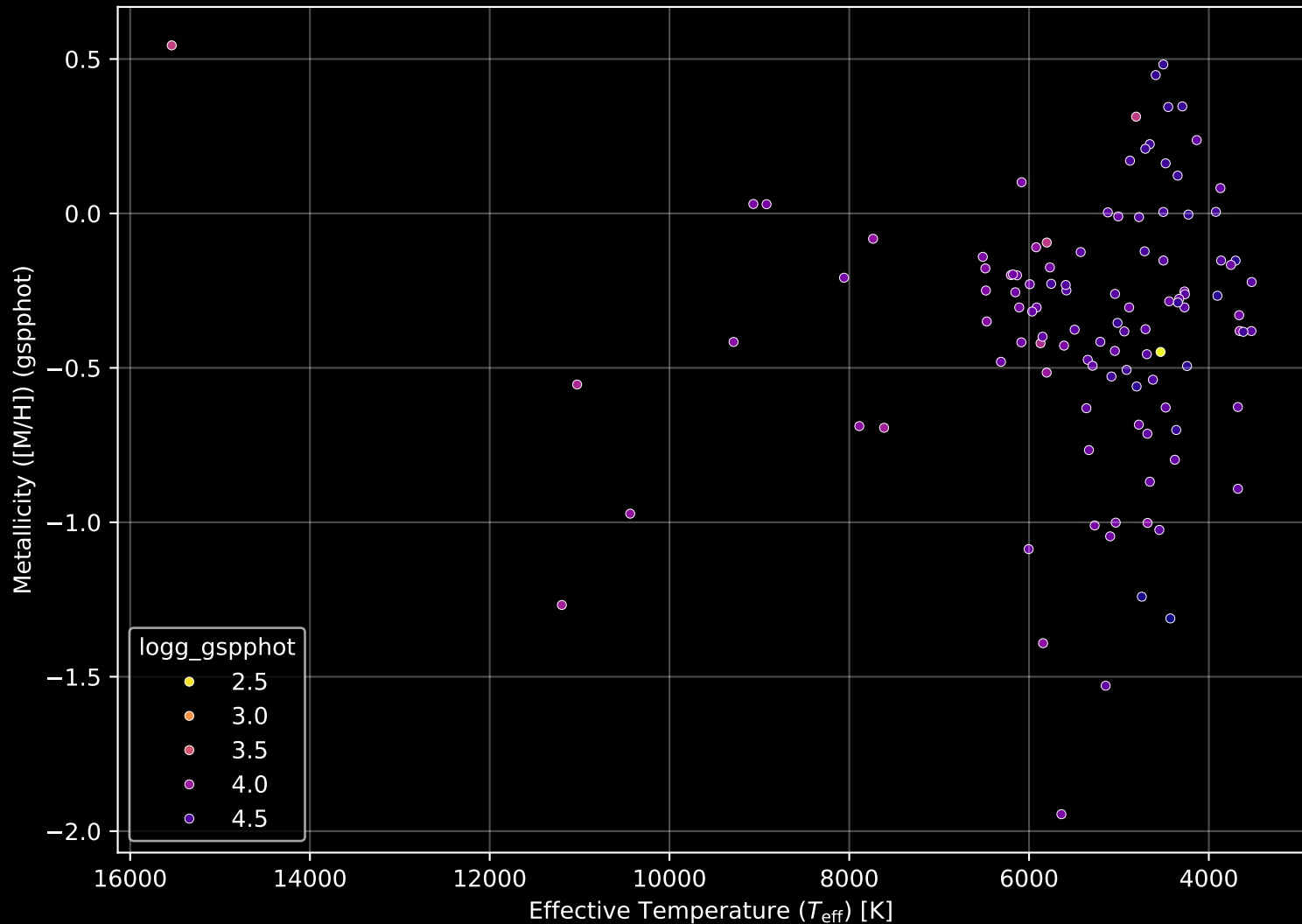
Gaia Cluster: [UPK_108] Stellar Population Parameters (n= 110)
