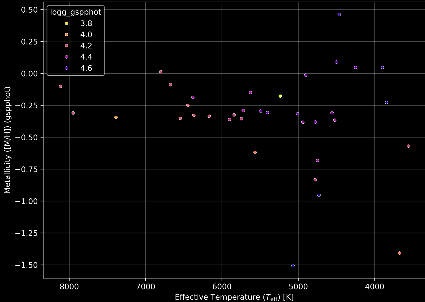
Gaia Cluster: [UPK_119] Stellar Population Parameters (n= 36)
