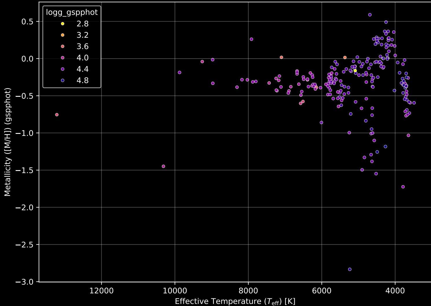
Gaia Cluster: [UPK_167] Stellar Population Parameters (n= 221)
